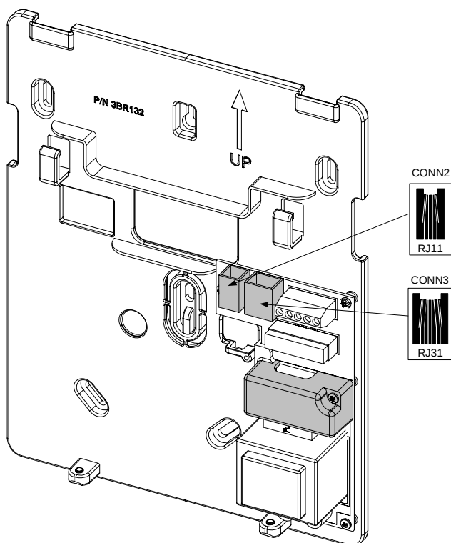
Figure 7 : Connecteurs de ligne téléphonique
