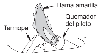
Figura 23 - Patrón incorrecto de la llama del piloto
