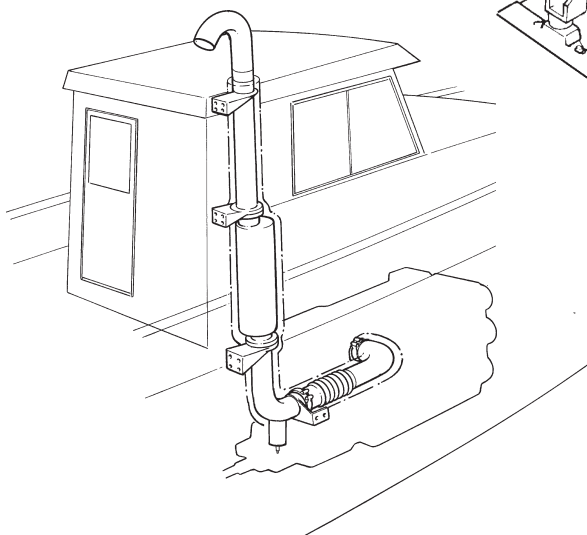
Système d'échappement sec
