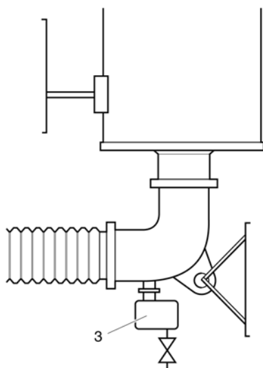
Exemple : Montage d'un collecteur d'eau de condensation pour les D16.
