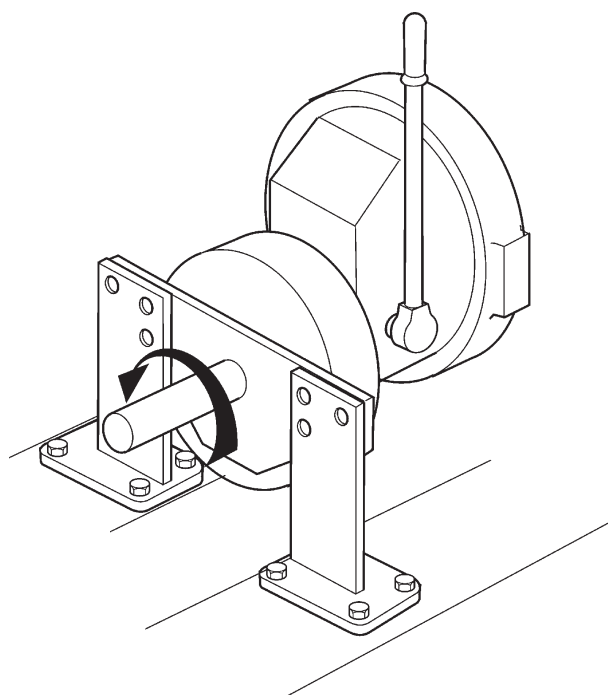
Prise de force avec réducteur, démultiplication 2,8:1. Sens de rotation : Sens anti-horaire. Dispositif de support inclus.
