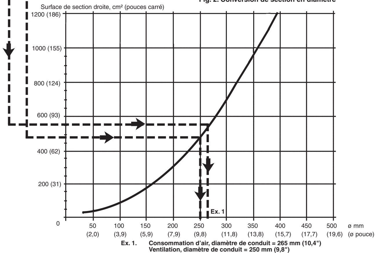
Fig. 2. Conversion de section en diamètre
