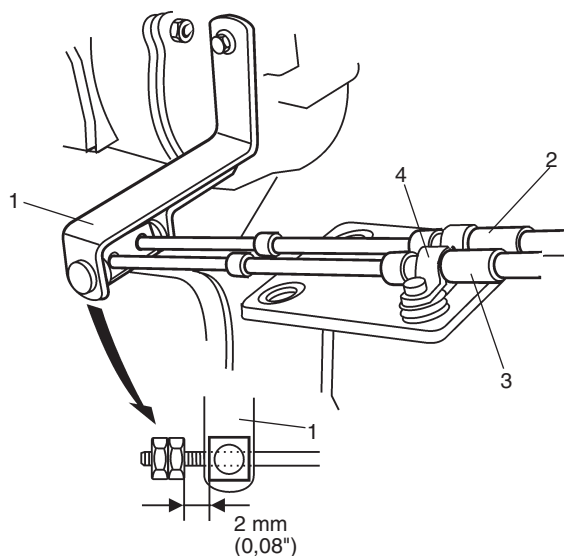
Branchement des câbles de commande d'accélérateur pour deux postes de commande
