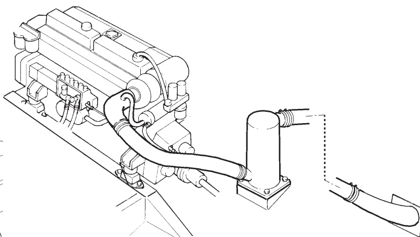
Système d'échappement à injection d'eau
