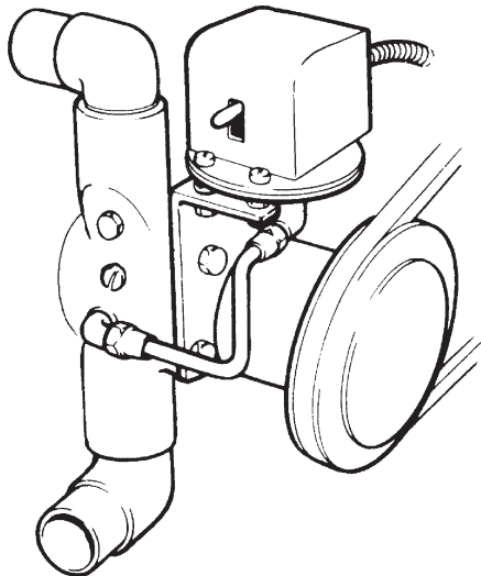
Pompe de cale (2"). Mise en service et arrêt électriques. Dépressiomètre pour désactivation automatique.
