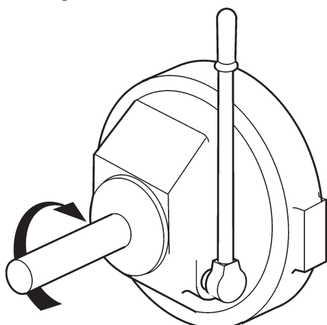
Prise de force, démultiplication 1:1. Sens de rotation : Sens horaire.
