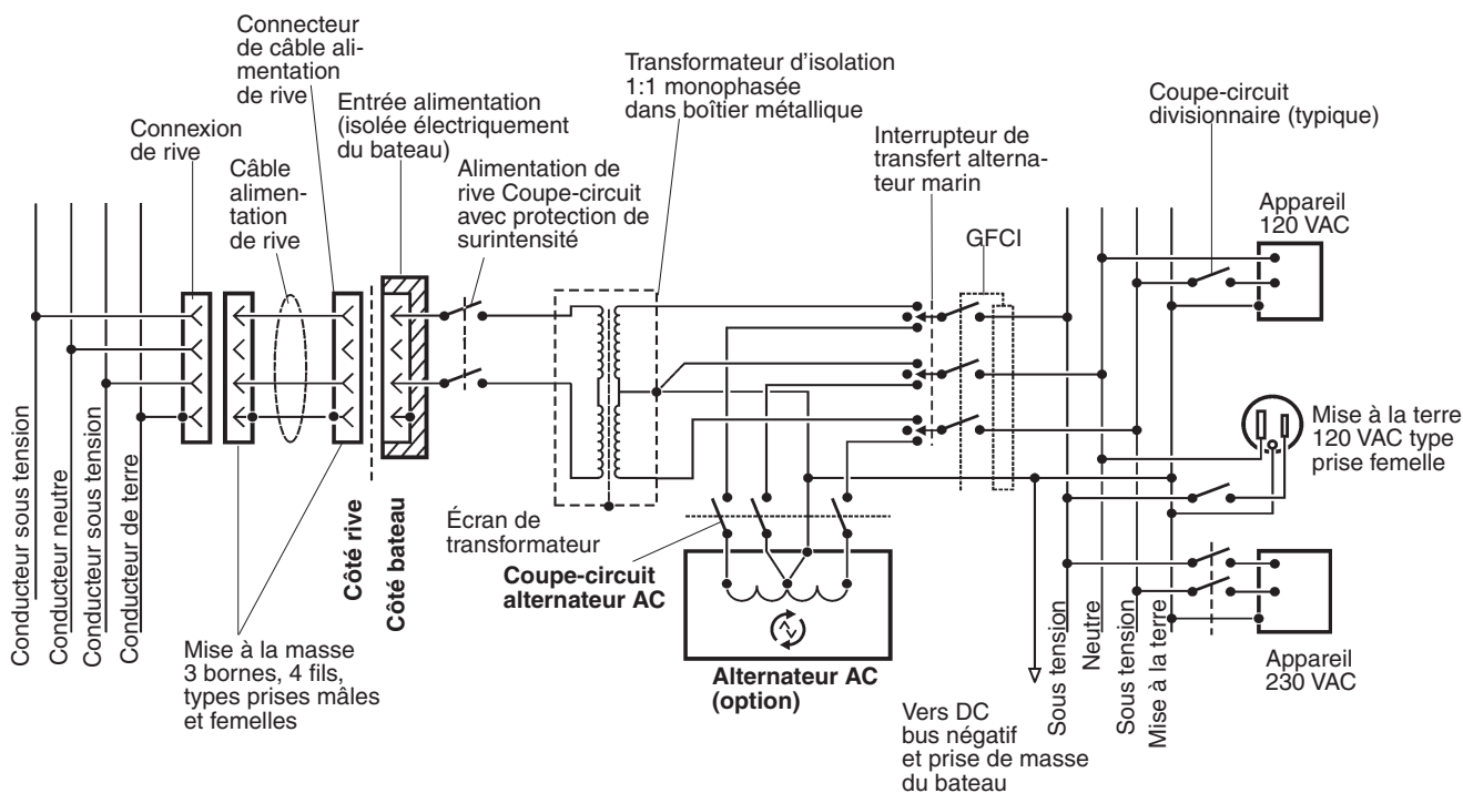
Figure 2 Monophasé, entrée 230 VAC, sortie 120 / 230 VAC
