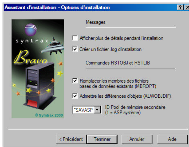
Figure 12: Options d'installation
