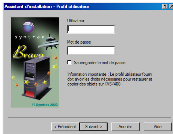
Figure 8: Profil utilisateur
