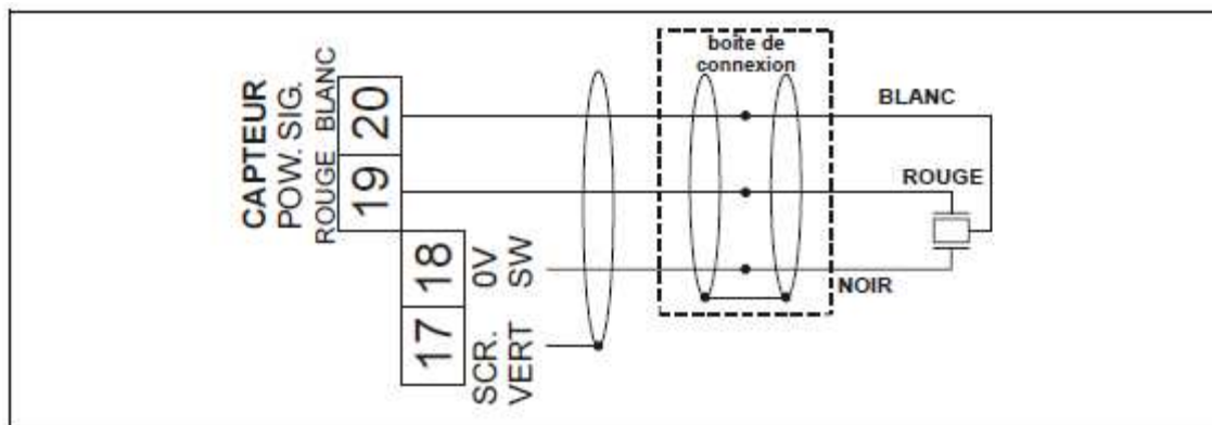
Fig. 6-3 Connexion d'un capteur ultrasonique de la série P
