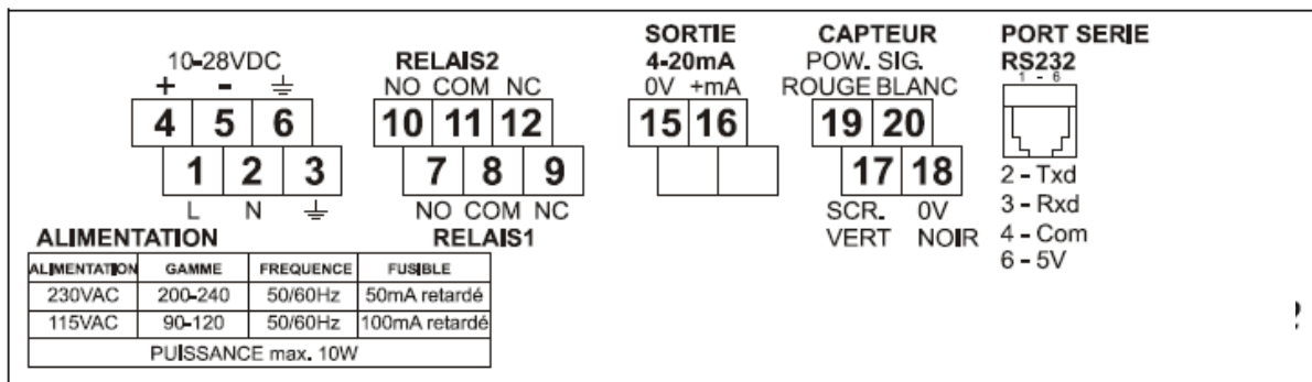
Fig. 6-2 Occupation des bornes du boîtier montage mural NM L-2
