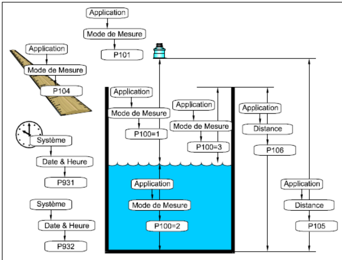
Fig. 6-8 Exemple d'application – mesure de niveau Paramètres de base
