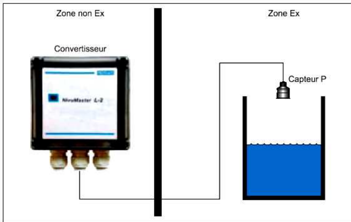
Fig. 6-4 Connexion en zone Ex
