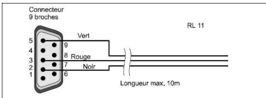
Fig. 6-5 Câble de liaison du NivuMaster vers un PC
