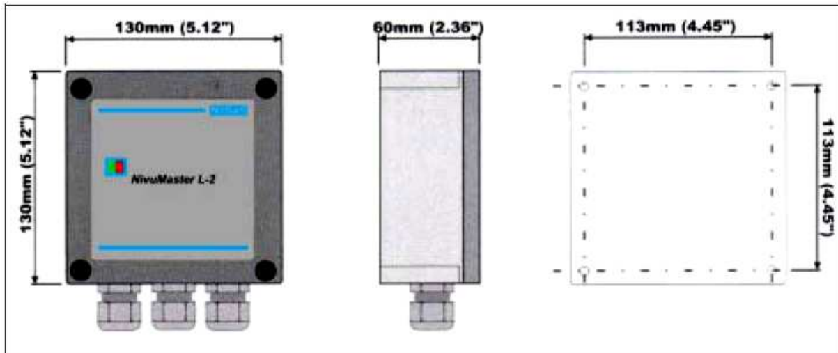
Fig. 6-1 Boîtier montage mural
