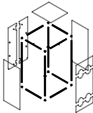
Bausatz Kälteisolierung
