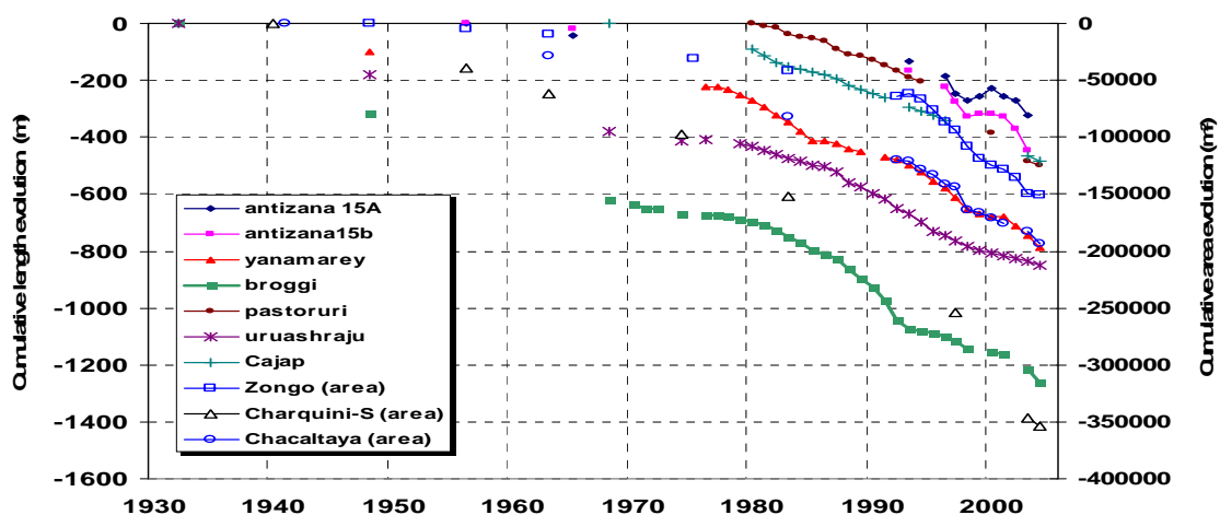
Figure 8. Evolution de la longueur ou de la surface de dix glaciers en Equateur (Antisana 15a and 15b), au Pérou (Yanamarey, Broggi, Pastoruri, Urushraju, Cajap) en Bolivie (Zongo, Charquini, Chacaltaya) entre 1930 et 2005. (Francou & Vincent, 2007).
