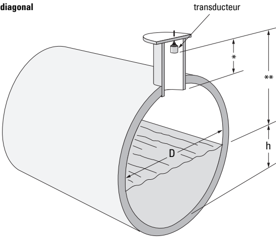
Profil diagonal
