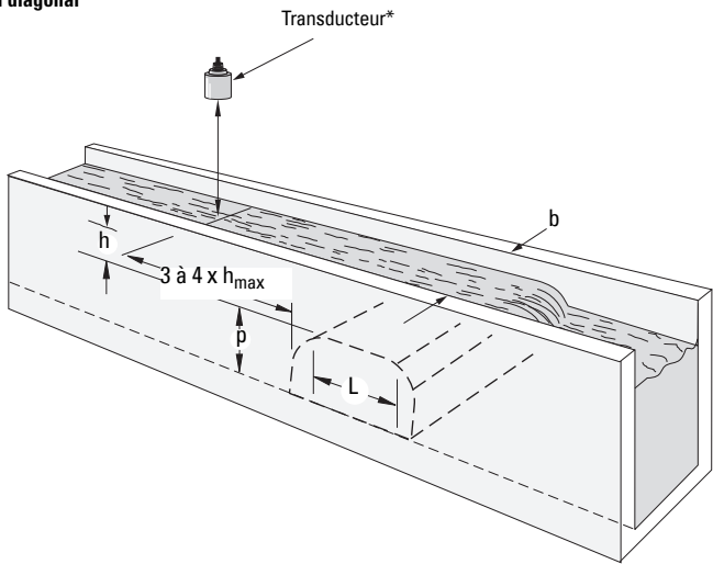
Profil diagonal
