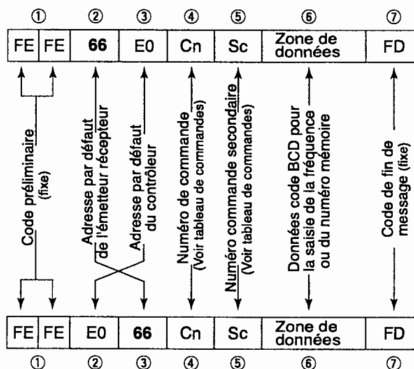
De l'IC-7400 vers le contrôleur
