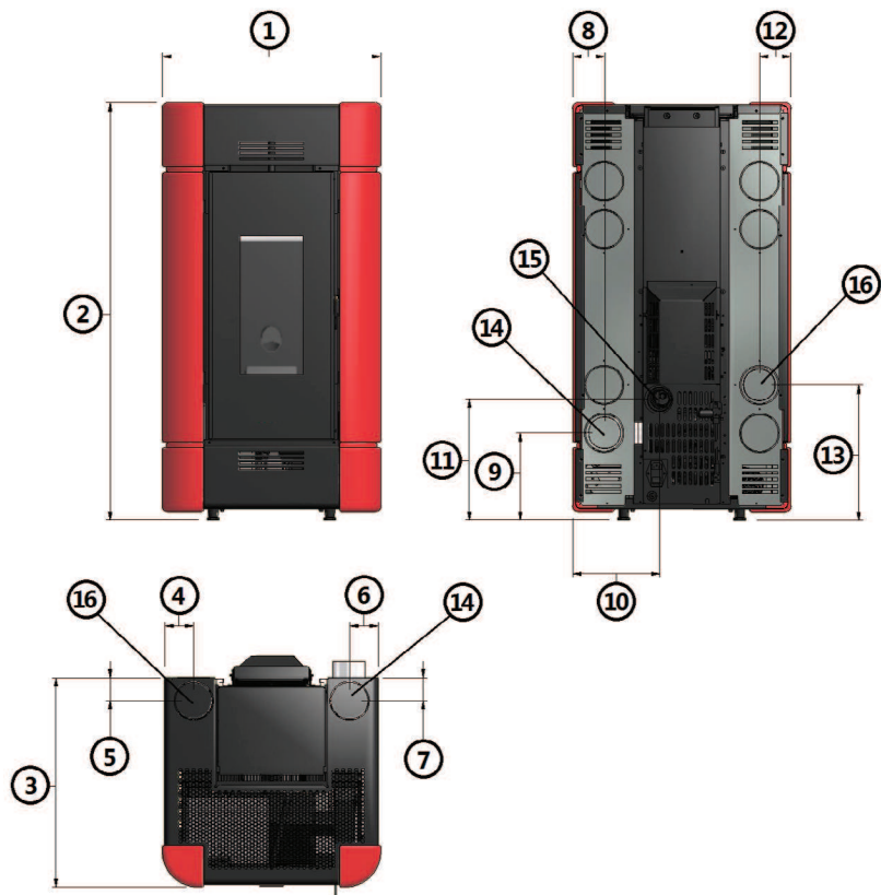
Fig. 13 - Dimensions générales: Sire Plus
