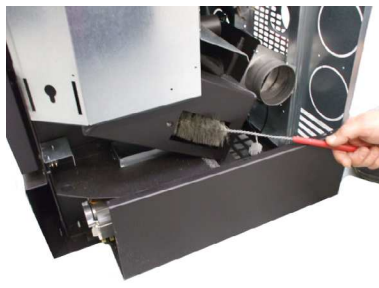
Fig. 56 - Nettoyage avec nettoie-pipes 2
