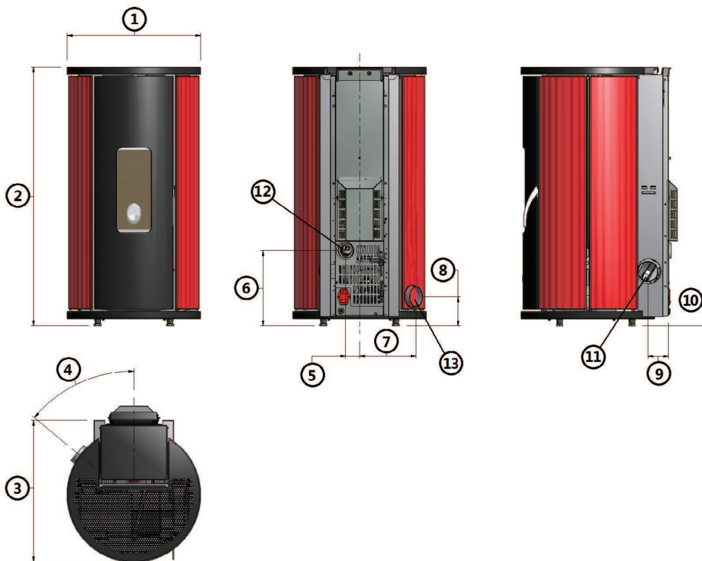
Fig. 15 - Dimensions générales: Sfera / Sfera Plus
