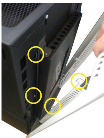
Fig. 17 - Assembler le panneau frontal
