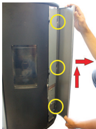
Fig. 51 - Sfera / Sfera Plus : décrocher les panneaux latéraux
