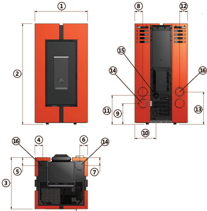
Fig. 14 - Dimensions générales: Doge Plus
