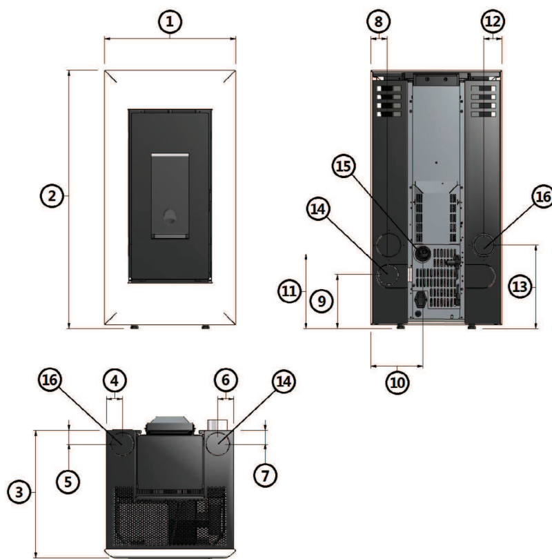
Fig. 12 - Dimensions générales: Vega
