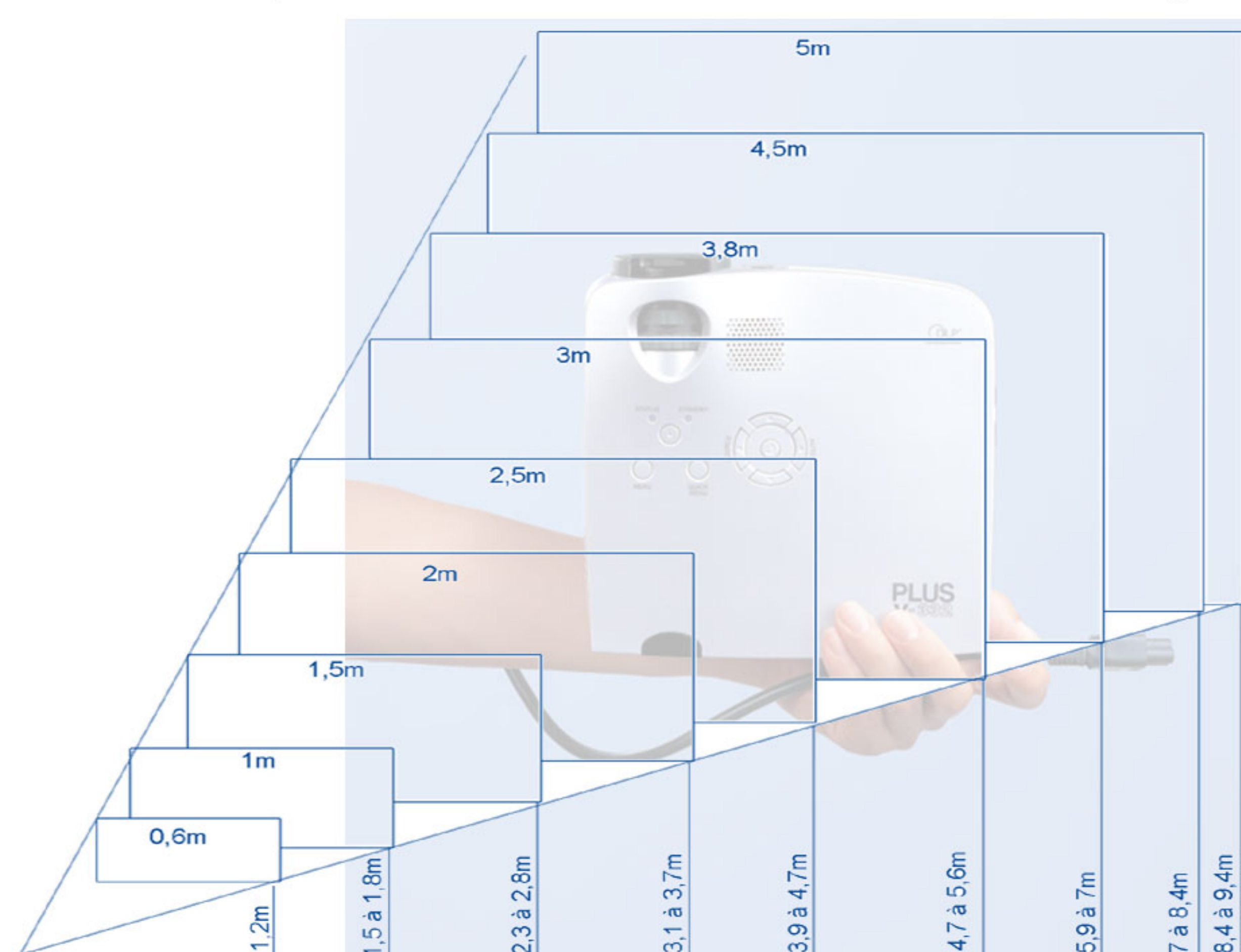
Taille d'écran et distances de projection du V339
