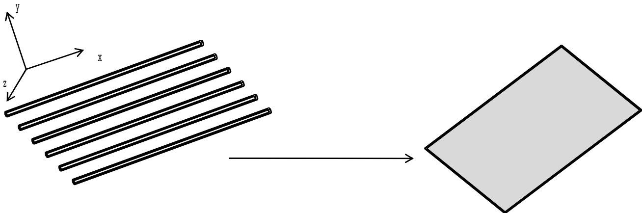
Figure 16.2-1: remplacement des armatures par une nappe équivalente
