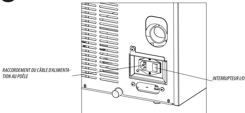
BRANCHEMENT ÉLECTRIQUE DU POÊLE.
