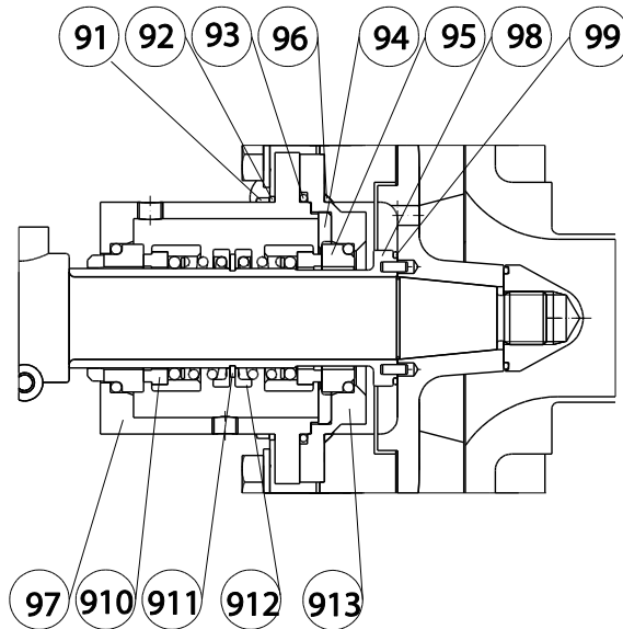
Figure 7 Garniture mécanique F11.
