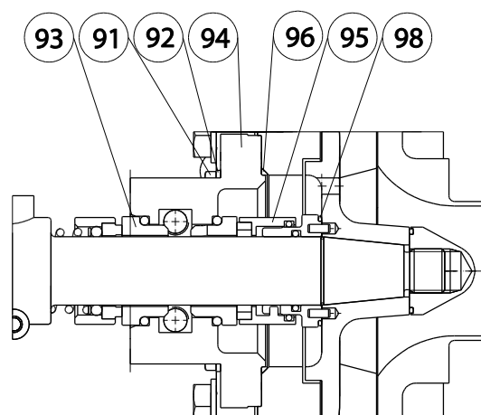
Figure 6 Garniture mécanique Q12.
