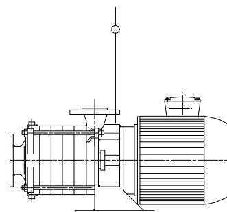
Groupe motopompe
