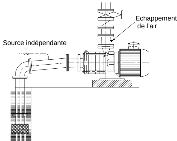
Amorçage pompe en aspiration avec clapet de pied
