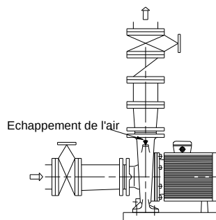
Amorçage d'une pompe en charge
