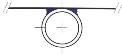
Figure 2 ter - Détail soudure du tube cuivre sur la tôle d'absorbeur des capteurs "SCHÜCOSOL K-S, K-S.1 et K-S.2"
