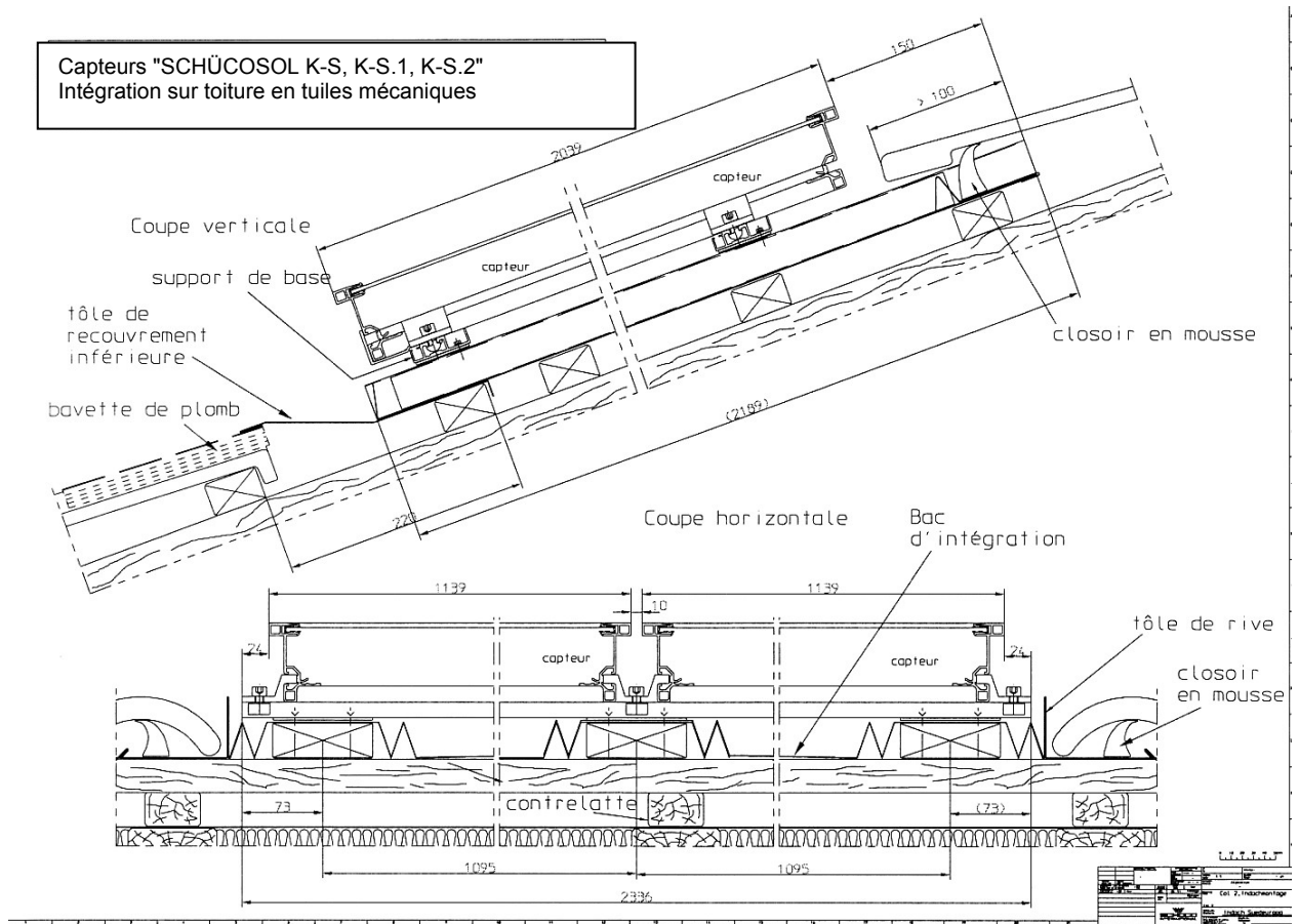
Figure 1.3 - Vue en coupe du montage des capteurs "SCHÜCOSOL K-S, K-S.1 et K-S.2" intégrés dans une toiture en tuiles mécaniques. Montage en vertical (ou en horizontal suivant le même principe). Voir également figure 1.6
