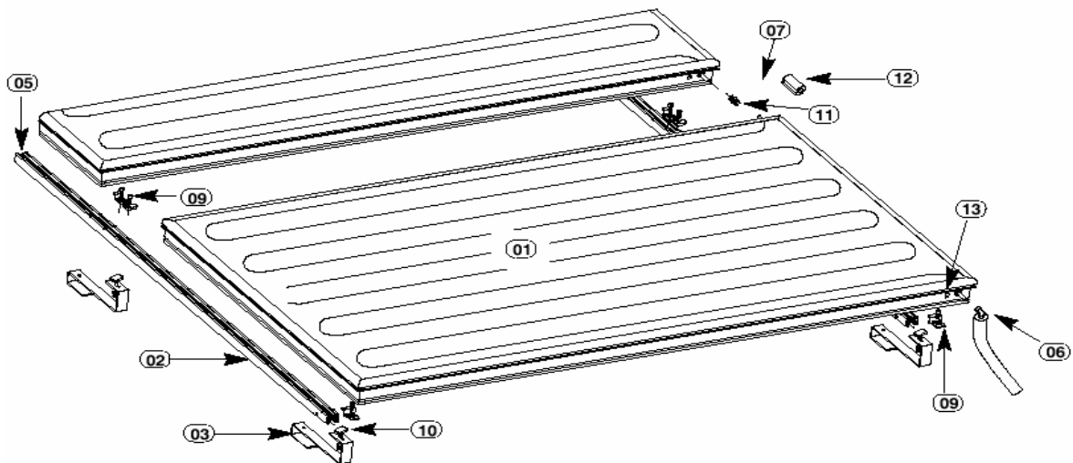
Figure 2.1 - Schéma d'ensemble du montage en appui sur toiture des capteurs "SCHÜCOSOL K-S"
