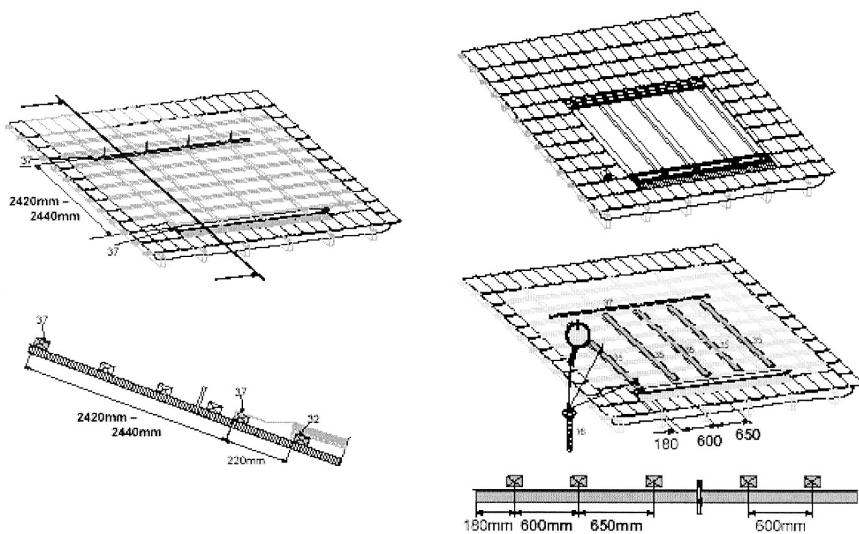
Figure 1.2 - Détail positionnement des lattes de support
