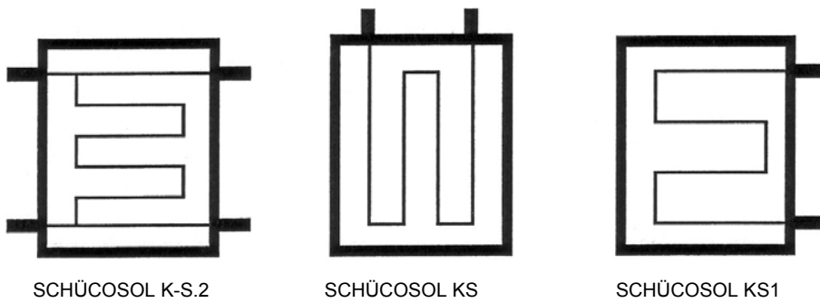
Figure 2 - Capteurs "SCHÜCOSOL K-S, K-S.1 et K-S.2" - Principe hydraulique des absorbeurs
