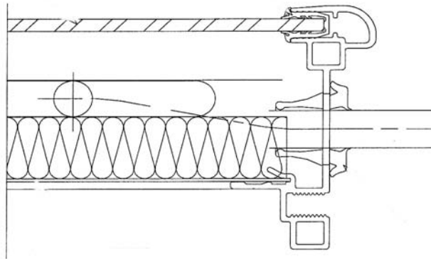
Figure 1 - Capteurs "SCHÜCOSOL K-S, K-S.1 et K-S.2" - vue en coupe
