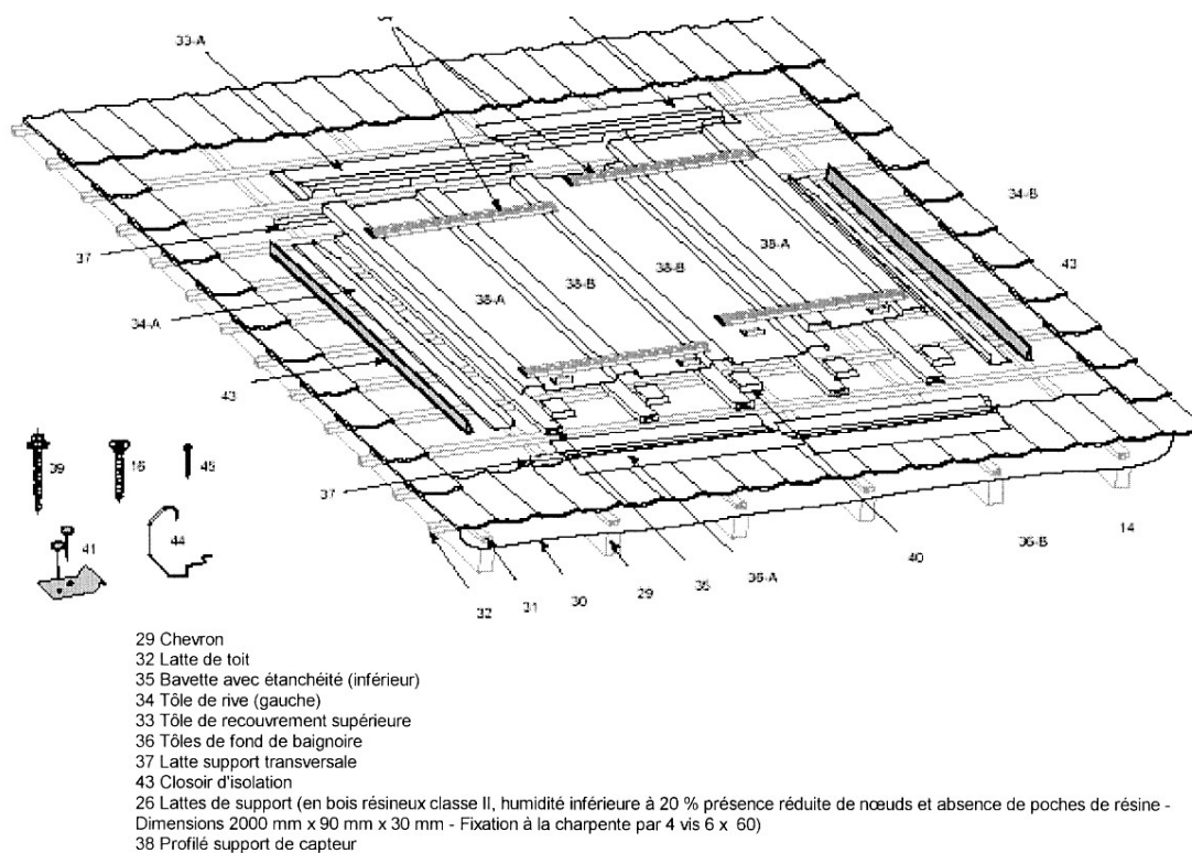
Figure 1.1 - Vue d'ensemble du montage
