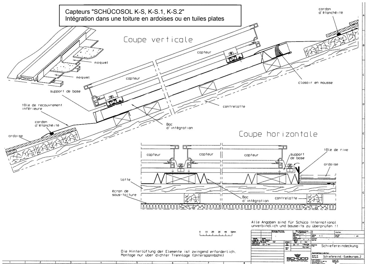
Figure 1.4 - Détails des raccords du montage des capteurs "SCHÜCOSOL K-S, K-S.1 et K-S.2" intégrés dans une toiture en tuiles plates ou en ardoises. Montage en vertical (ou en horizontal suivant le même principe). Voir également figure 1.6
