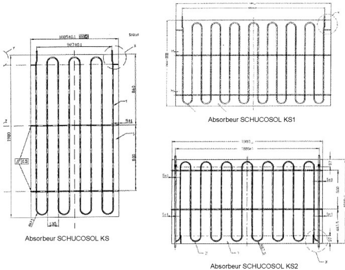
Figure 2 bis - Capteurs "SCHÜCOSOL K-S, K-S.1 et K-S.2" - Vue en plan des absorbeurs
