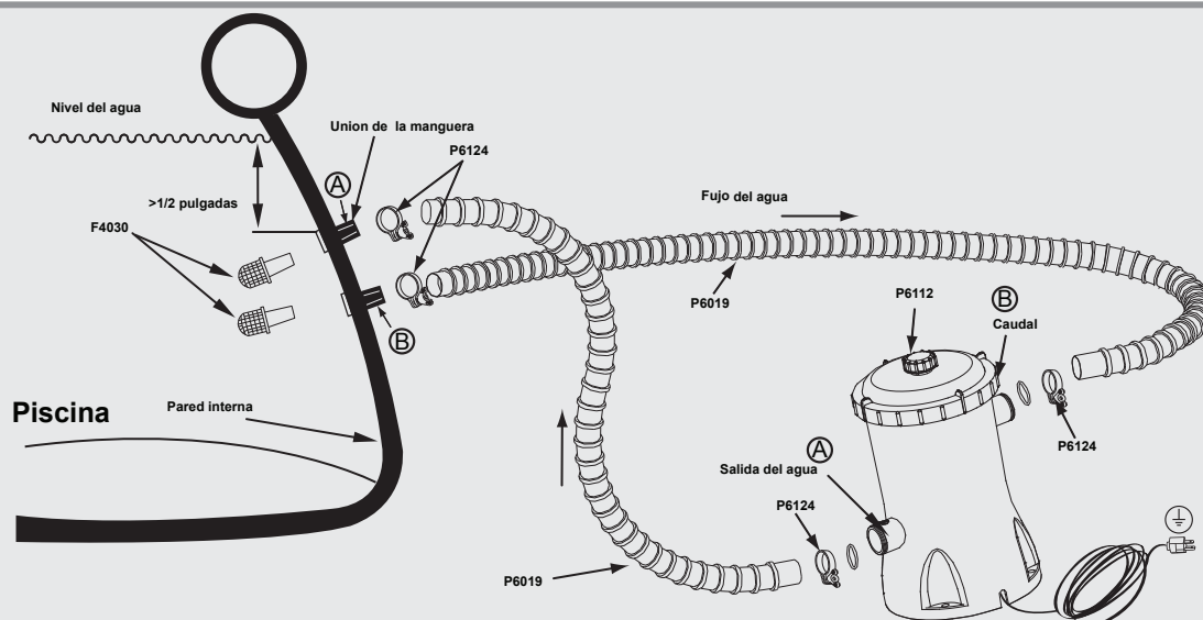
Ilustración (no en escala) de la piscina y de la bomba de filtro HOWLIAR™
