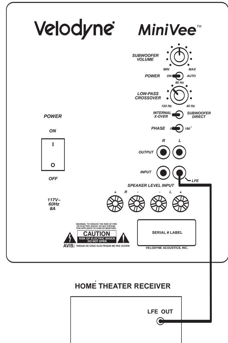
Figure 1. Installation à l'aide des entrées LFE de niveau de ligne
