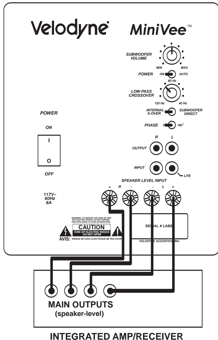
Figure 3. Installation à l'aide des entrées de niveau haut-parleur
