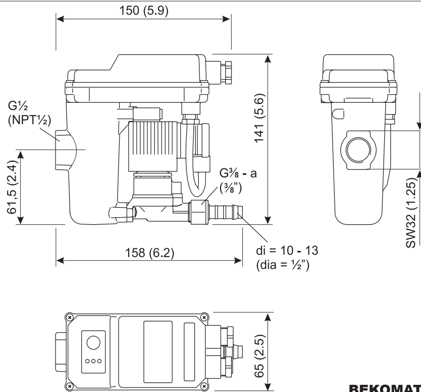
BEKOMAT® 12 BEKOMAT® 12 CO
