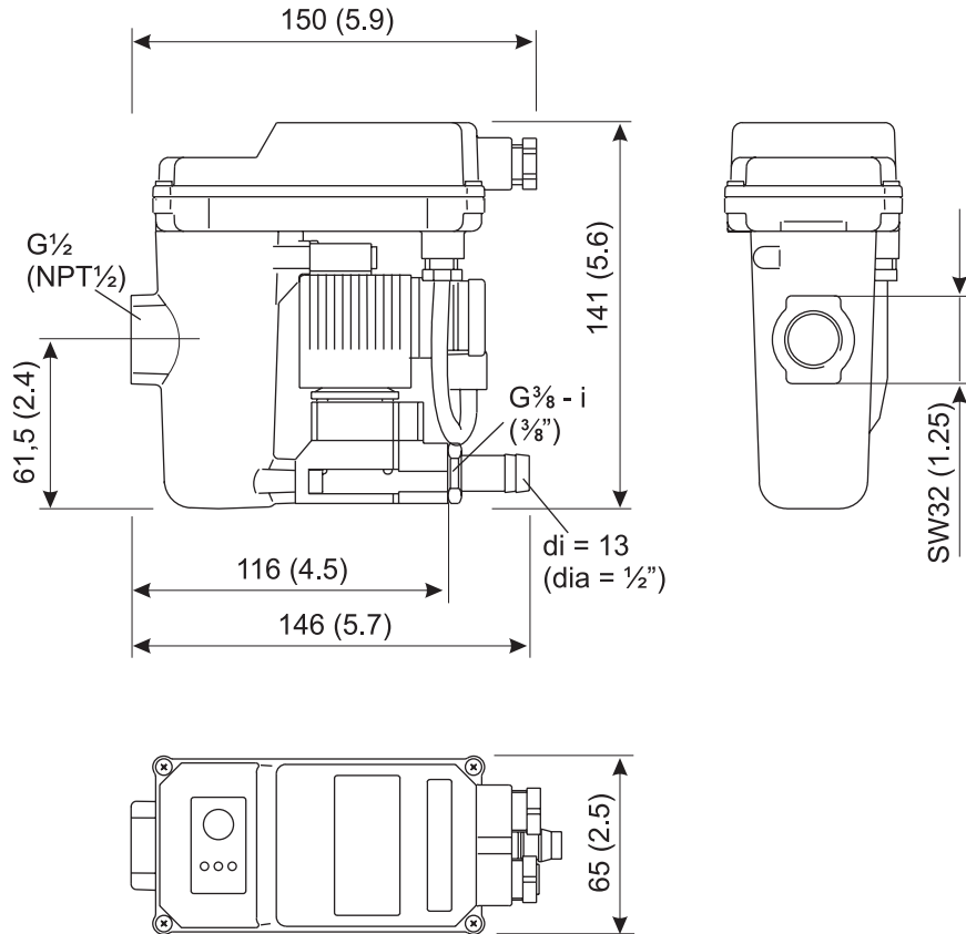
BEKOMAT® 12 CO PN63
