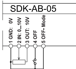
Contact ouvert = Arrêt Contact fermé = Marche
