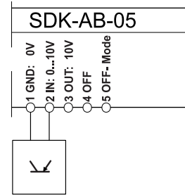
Commande avec source de courant absorbé (p. ex. EIB)
