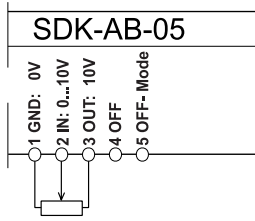
Commande avec potentiomètre
