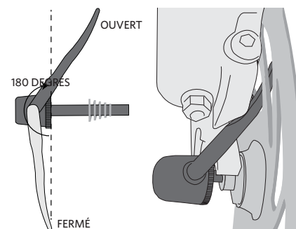
Figure 1. Lever de blocage rapide ouvert au-delà de 180 degrés
