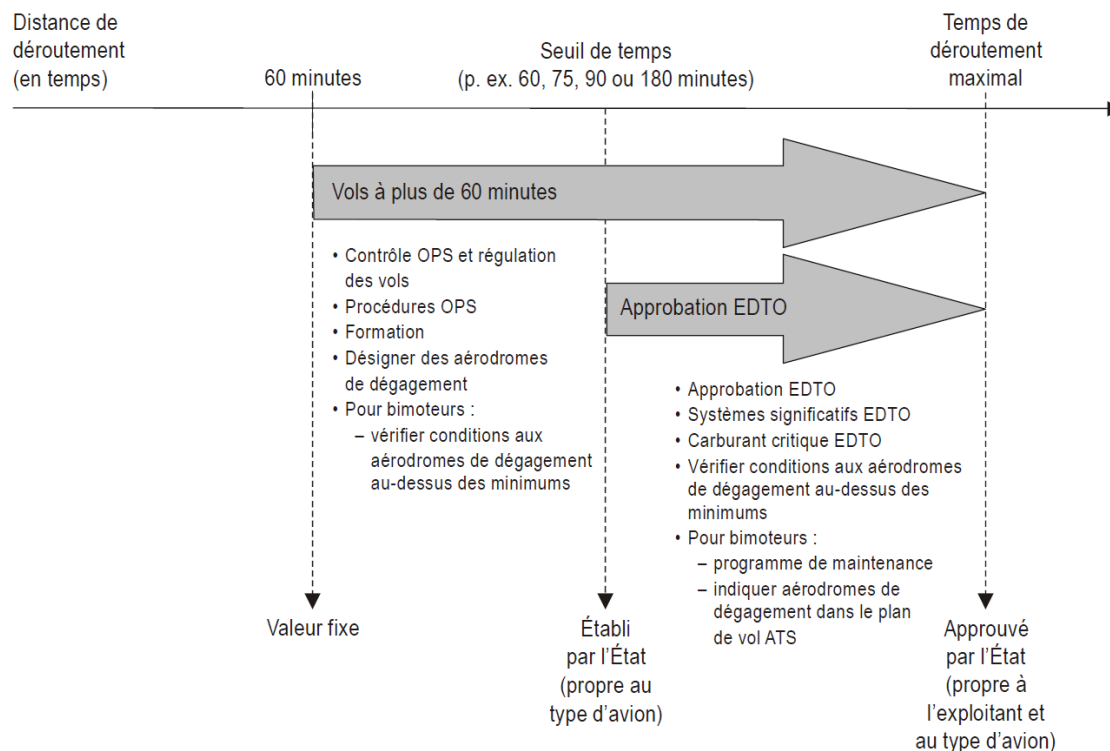
Figure 1. Représentation graphique générique de l'exploitation EDTO
