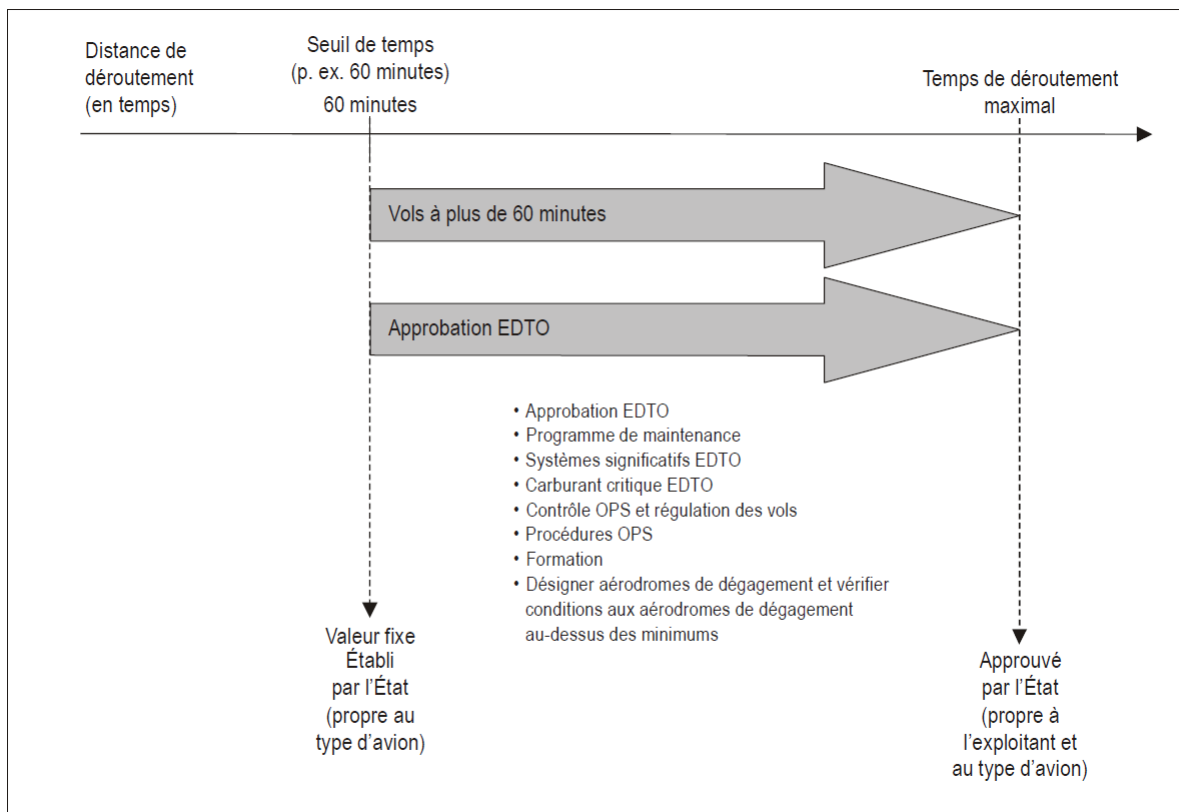
Figure 7. Représentation graphique générique de l'exploitation EDTO d'avions à deux turbomachines
