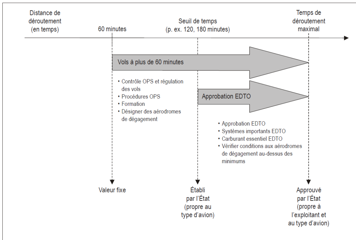
Figure 4. Représentation graphique générique de l'exploitation EDTO d'avions équipés de plus de deux moteurs
