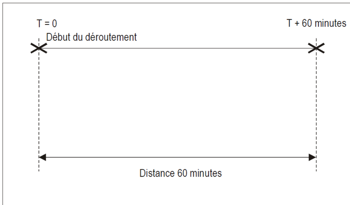
Figure 3. Distance 60 minutes — Avions équipés de plus de deux turbomachines
