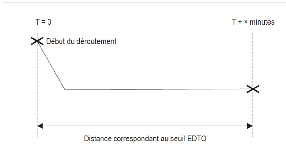
Figure 8. Seuil de distance — Avions équipés de deux turbomachines
