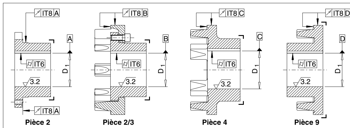
Fig. 4 : Alésage fini
