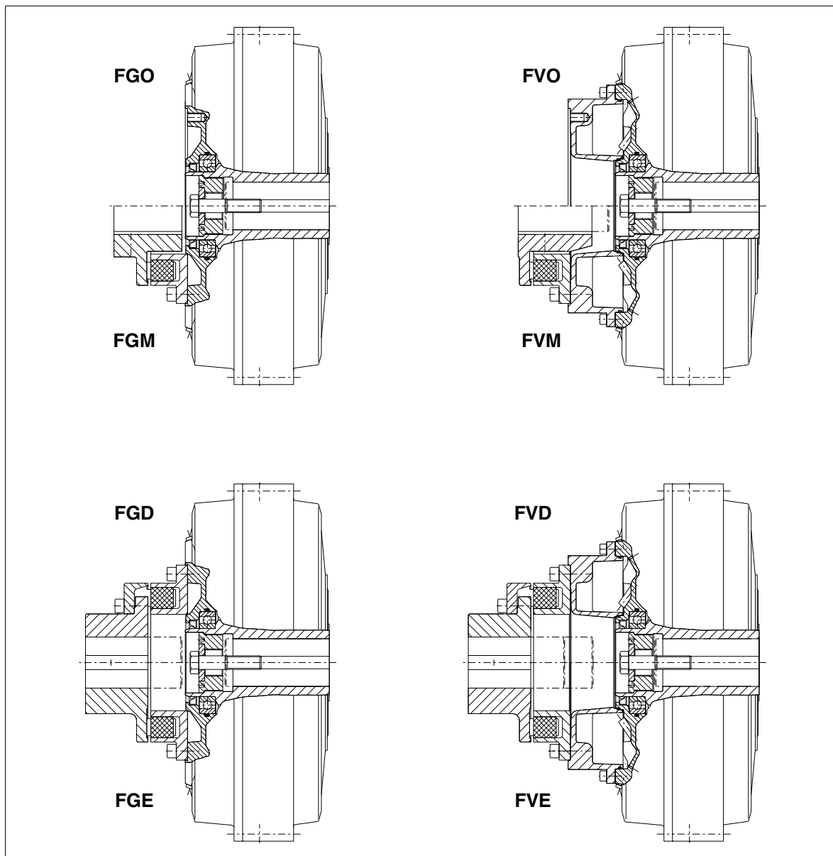
Fig. 1 : Types d'accouplement
