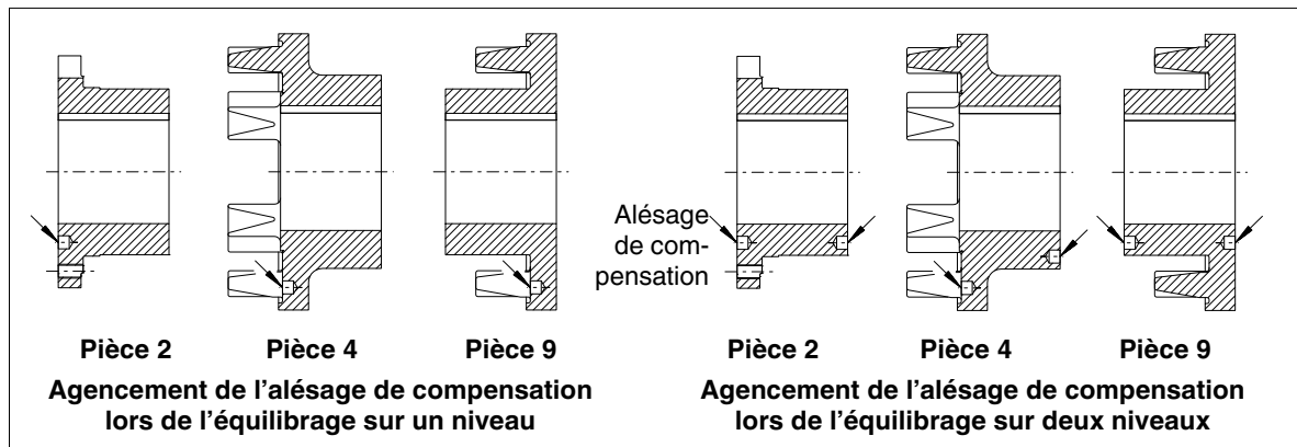
Fig. 7 : Équilibrage
