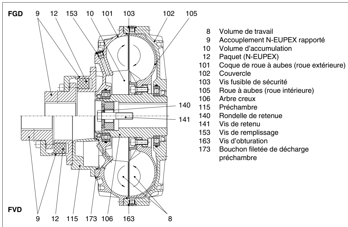
Fig. 3 : Description générale des séries "FG." et "FV."
