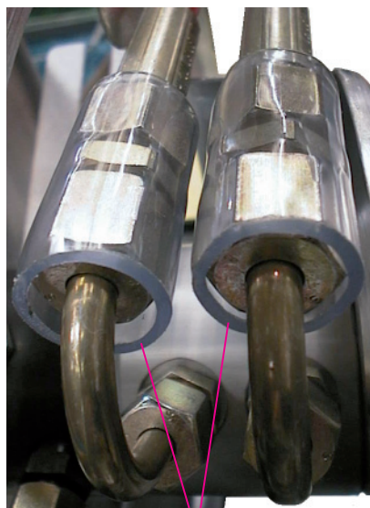
Tuyau de protection
