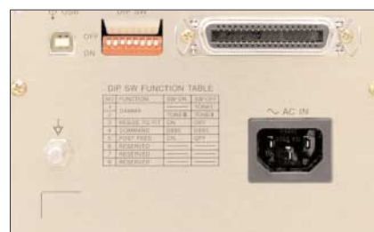
Panneau arrière
