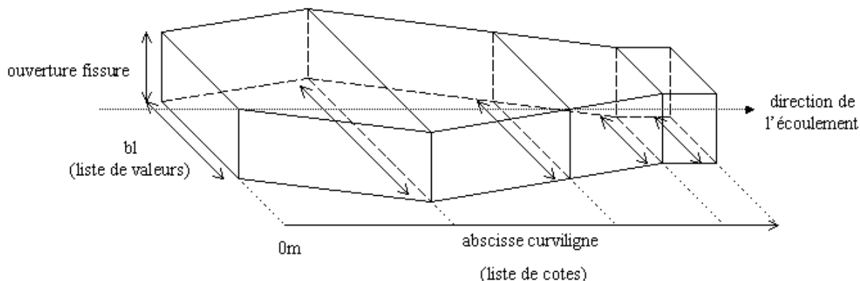
Figure 3.14.4-a: Représentation de la fissure
