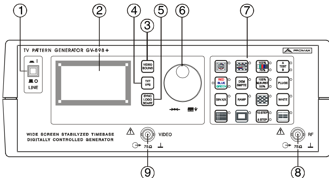
Figure 2.- Panneau avant
