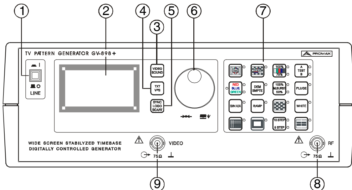
Figura 2.- Panel frontal
