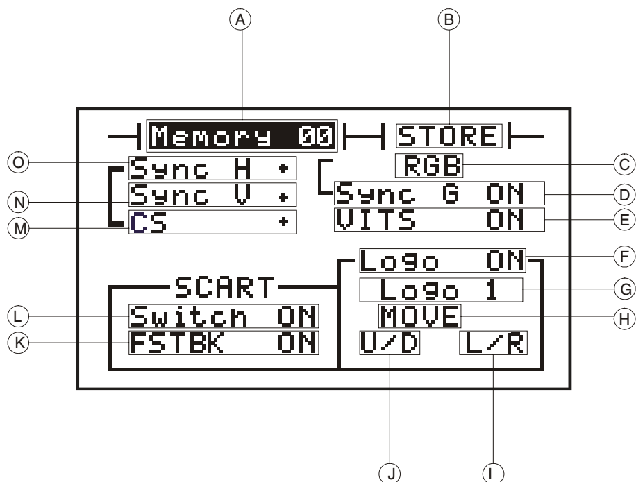
Figura 7.- Ejemplo de display del menú de configuración SYNC-LOGO-SCART
