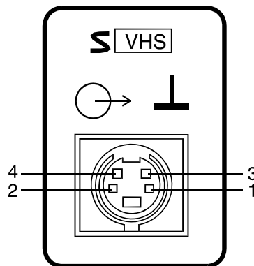
Figure 8.- Connecteur S-VHS
