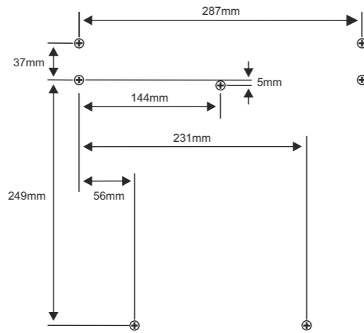
Bohrungsvorbild
