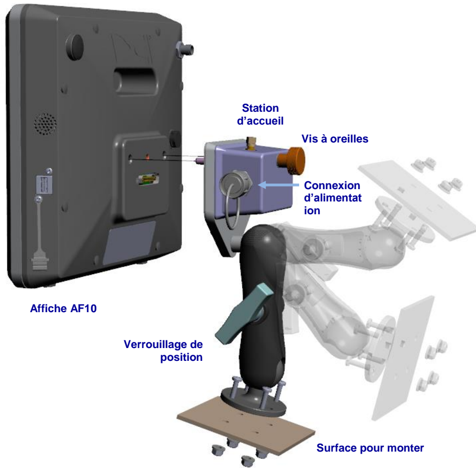
Image explosé d'AF10
