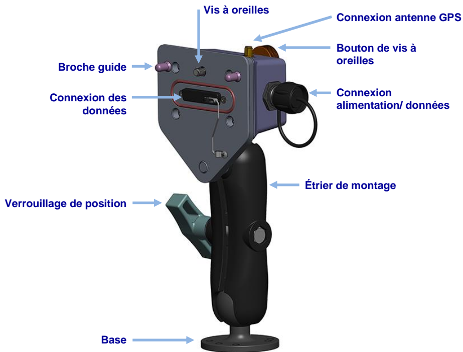
La station d'accueil de l'appareil de forage AF10
