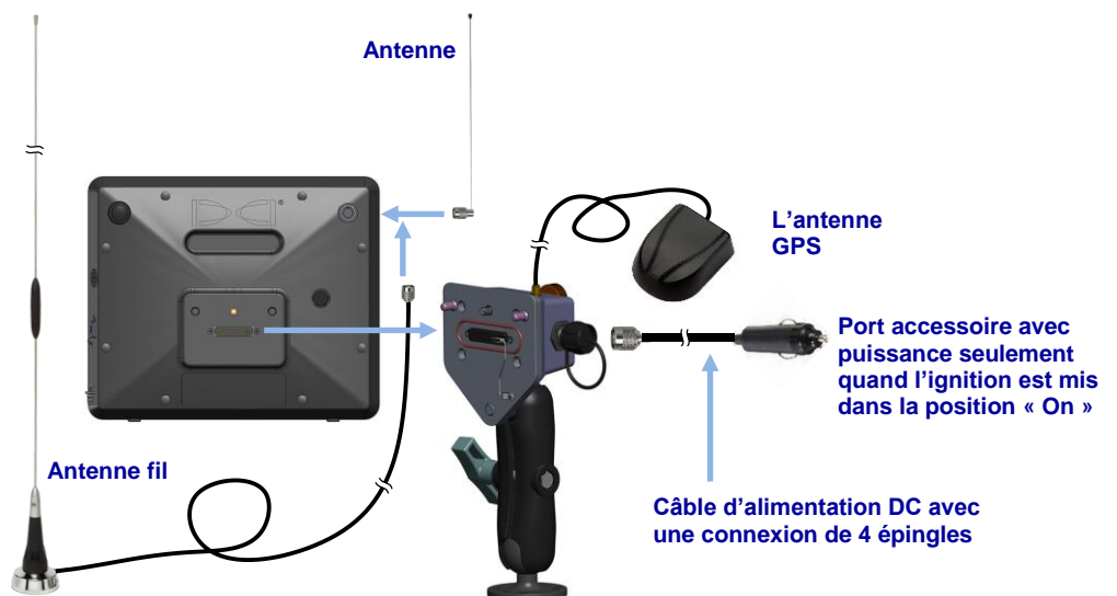
Connexions de câblage (montré aussi est l'antenne fil optionnel)
