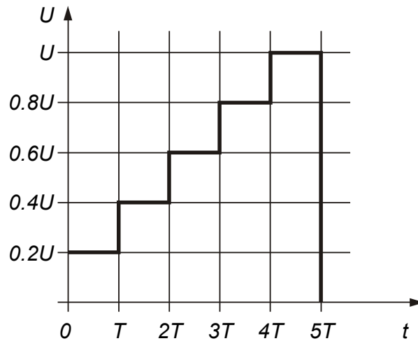
Schéma 24. Tension d'essai incrémentale
