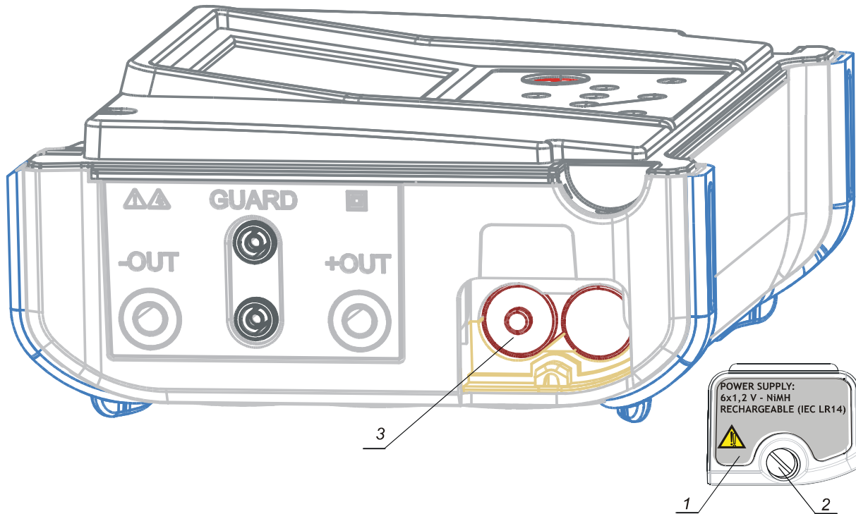
Schéma 32. Insertion des batteries
