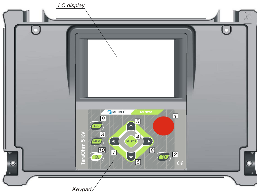
Schéma 1. Panneau avant
