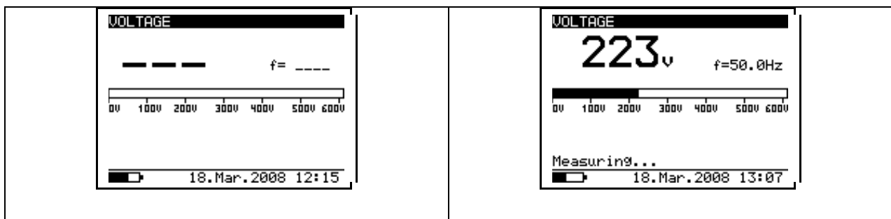
Schéma 10 Mesure de tension
