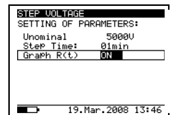
Schéma 26. Menu de réglage de la mesure de tension par pas.
