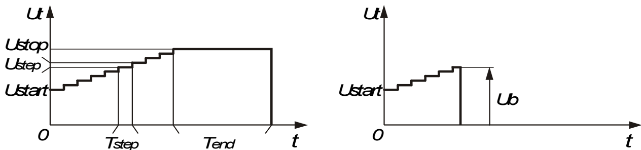
Schéma 28. Présentation de la tension d'essai sans rupture (à gauche) et avec rupture (à droite).
