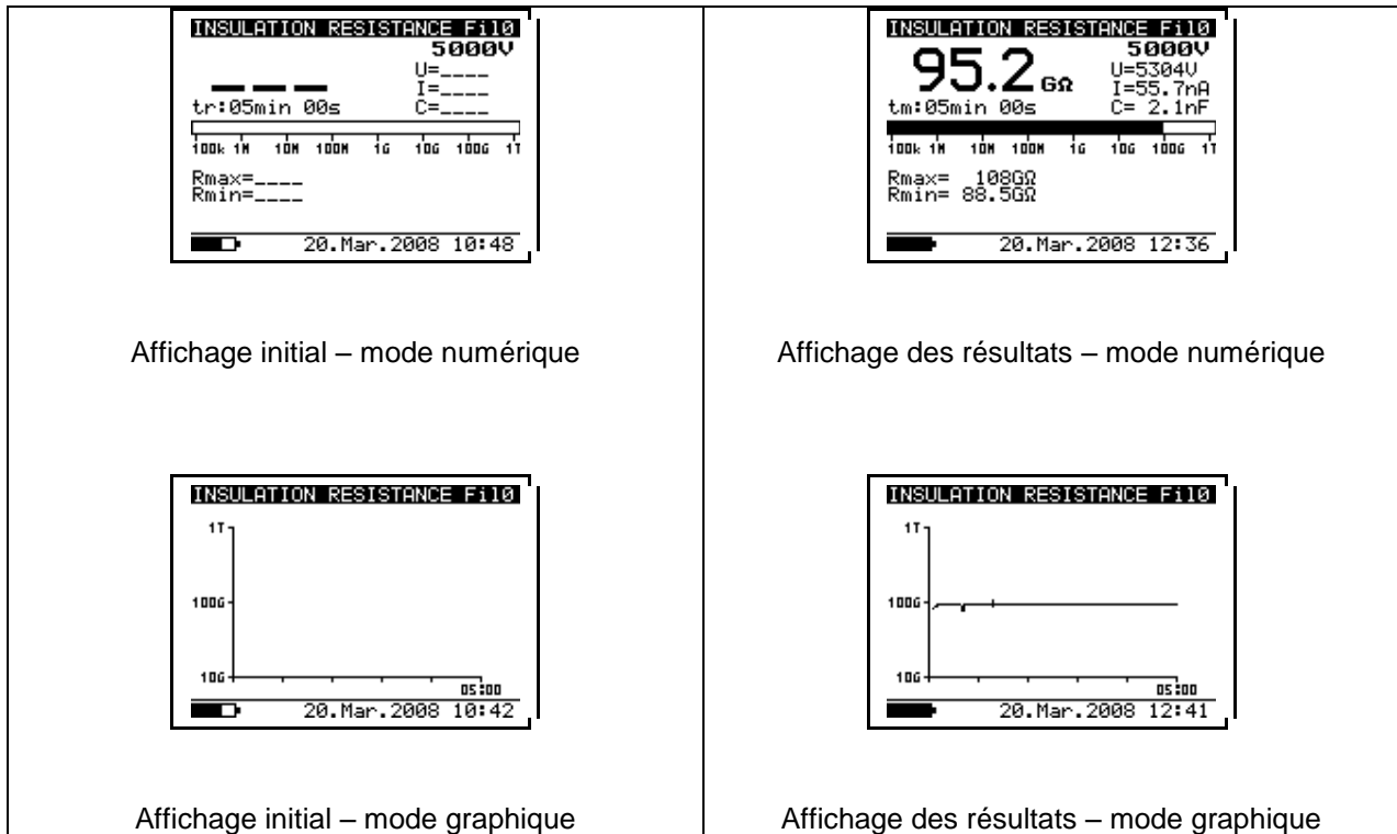
Schéma 12. Mode numérique ou graphique – Graphe R(t) activé
