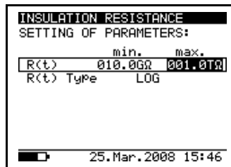
Schéma 15. Menu de réglage du Graphe R(t)
