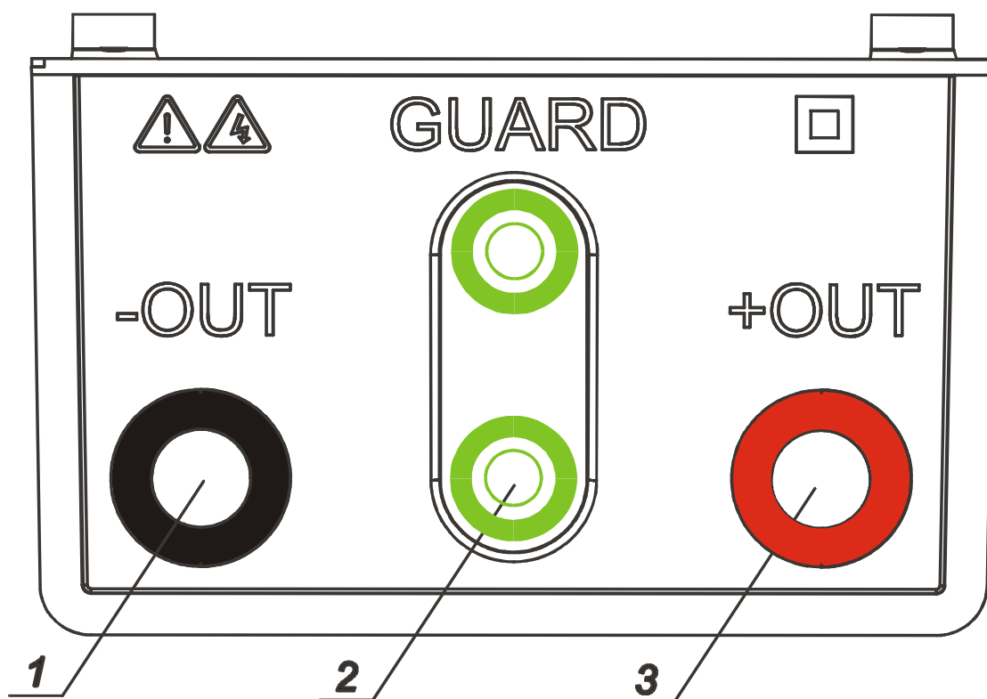
Schéma 2. Connecteurs des cordons de mesure.
