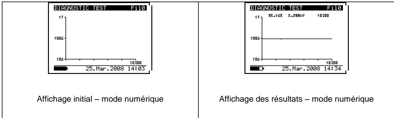
Schéma 17. Affichage des différents états du test de Diagnostic Graphe R(t) activé
