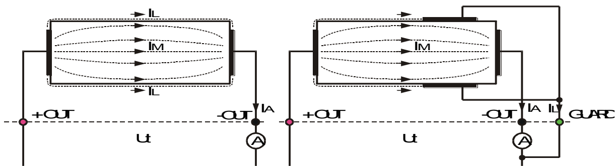
Schéma 9. Connexion d'un dispositif de garde à l'objet mesuré
