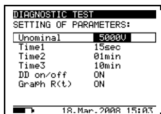
Schéma 18. Menu de configuration pour le test de Diagnostic
