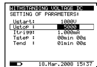
Schéma 30. Menu de réglage pour la Tension de résistance
