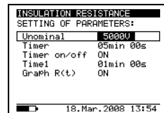
Schéma 13. Menu de Réglage pour une mesure de résistance d'isolement.
