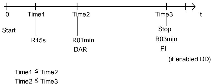
Schéma 19. Relation entre les minuteurs
