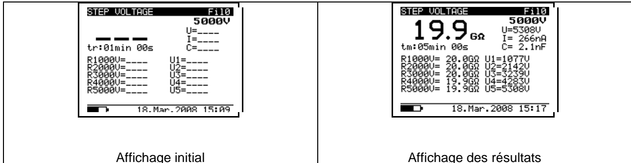
Schéma 22. Affichage des différents états de la fonction Echelon de Tension Graphe R(t) désactivé
