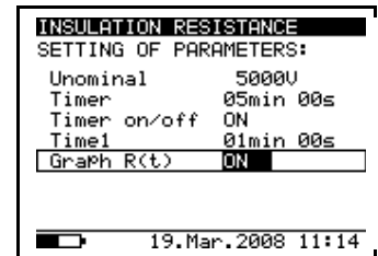
Schéma 14. Menu de réglage pour une mesure de résistance d'isolement
