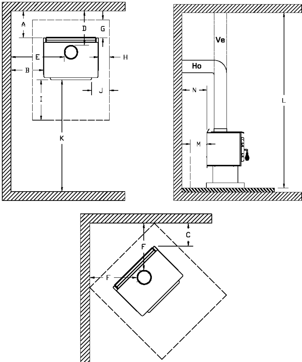
Figure 2 : Dégagements aux matériaux combustibles et protection de plancher
