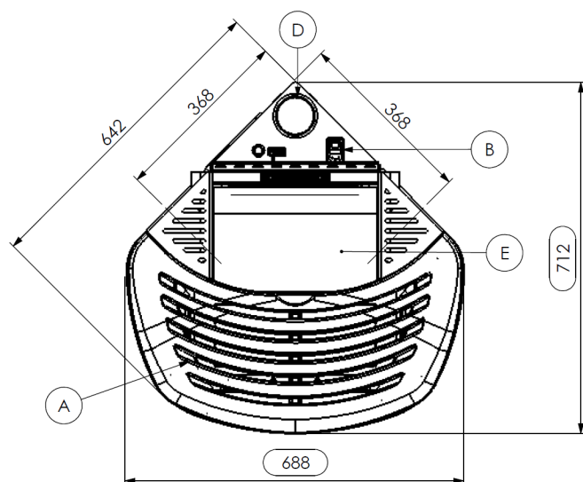
Ingombri stufa pellet MIMOSA CAN.
