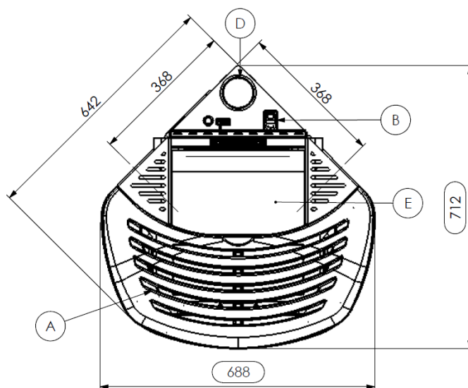
Medidas de la estufa de pellets MIMOSA CAN.
