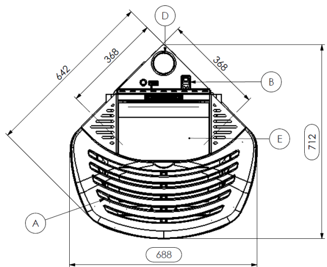
Abmessungen Pelletofen MIMOSA CAN .
