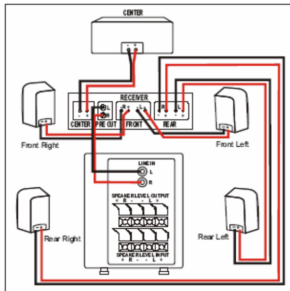
Raccordement de bas niveau
