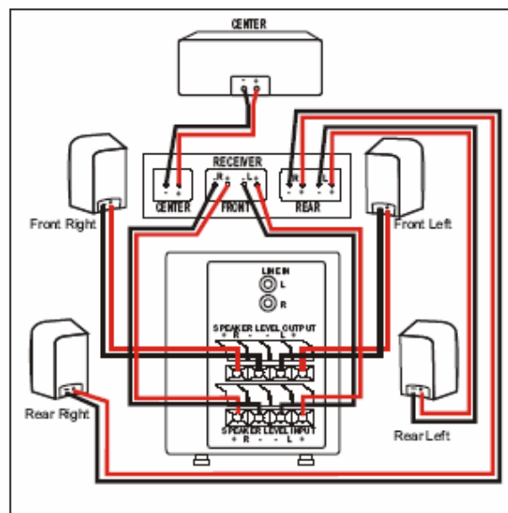
Raccordement de haut niveau
