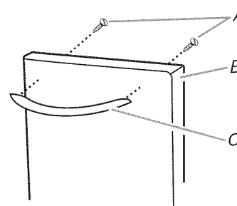
A. 2 vis insérées dans les trous, depuis l'intérieur du tiroir B. Partie supérieure du tiroir C. Poignée montée sur la façade du tiroir
