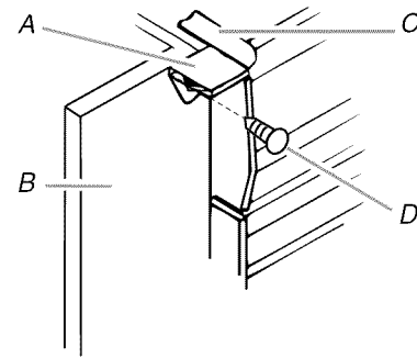
A. Agrafe de montage (fournie) B. Armoire C. Bride de retenue D. Vis de montage (fournie)
