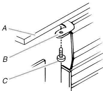
A. Comptoir B. Bride de retenue C. Vis de montage (fournie)
