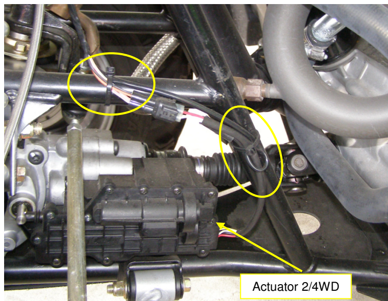
Photo 1: Cheminement câblage corrigé Verlegung der Verkabelung 2/4WD Stellmotor
