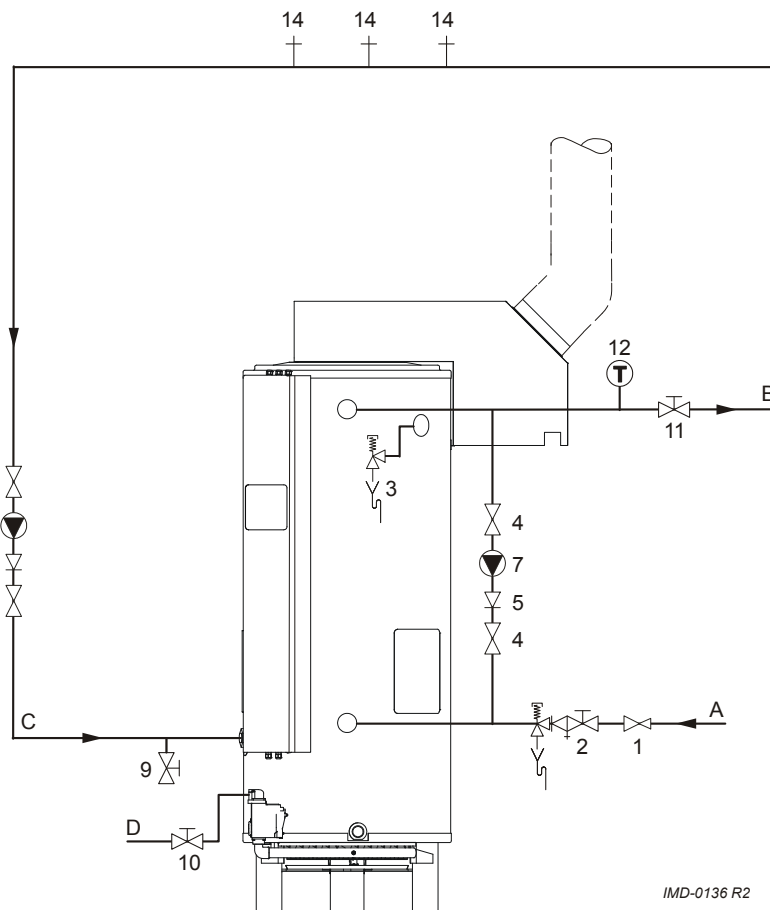
Schéma de raccordement
