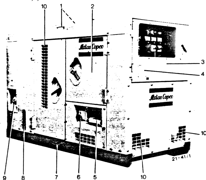
Fig. 2. QAS40
