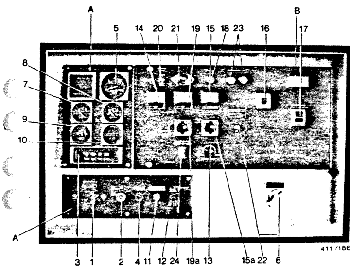
Fig. 8. QAS125 et -150
