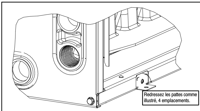
Figure 4 – Installation horizontale vers la gauche
