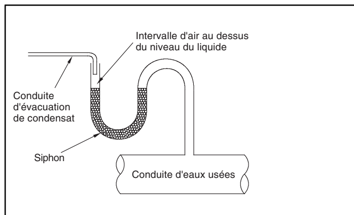
Figure 6 – Évacuation des condensats vers la conduite d'eaux usées
