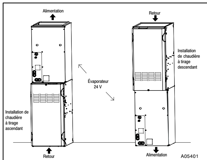
Figure 1 – Orientation adéquate du support du serpentin sur la chaudière
