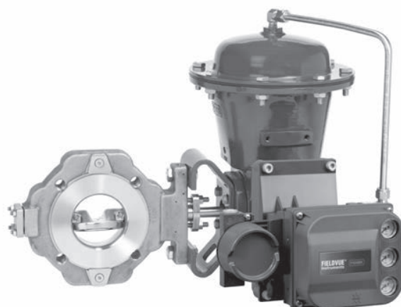
Figure 1. Vanne 8580 de Fisher avec actionneur 2052 et contrôleur numérique de vanne DVC6200
