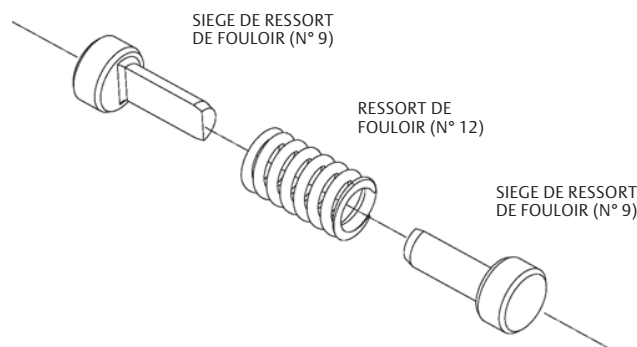
Figure 8. Ensemble ressort de fouloir-siège de ressort
