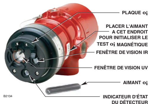
Figure 2—Vue de Face du X5200
