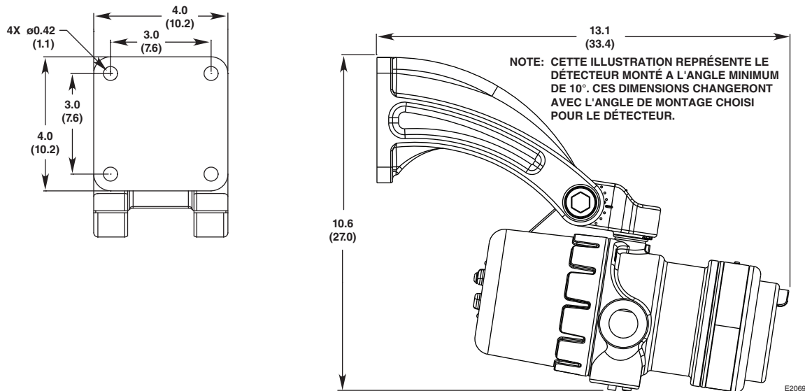
Figure 3—Dimensions du Support de Montage à Rotule Q9033 avec Collier de Fixation (cm) (Voir la Figure 1 pour l'Orientation Correcte du Détecteur)
