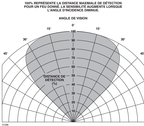
Figure 15—Cône de Vision du Détecteur
