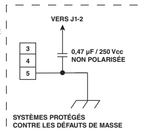
Figure 9—Système Type, Détecteurs X5200 Câblés sur un Contrôleur R7495
