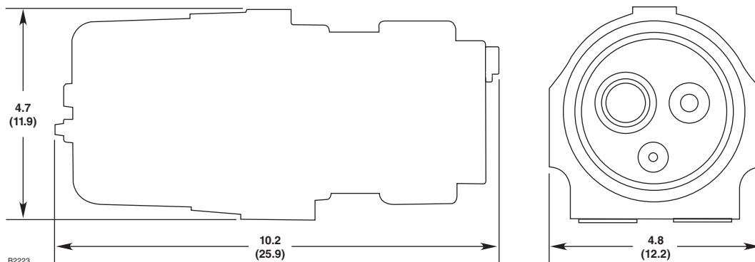
Figure 16—Dimensions du X5200 en cm
