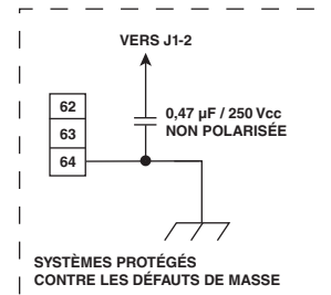
Figure 7—Système Type, Détecteurs X5200 Câblés sur un Contrôleur R7404 avec Star Logic
