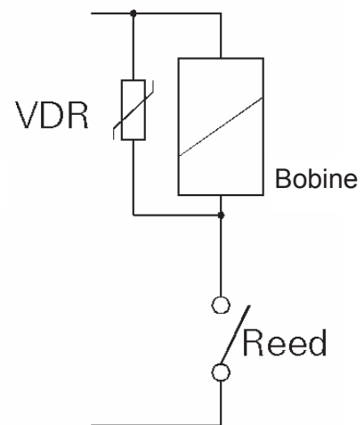
Alimentation Courant Alternatif
