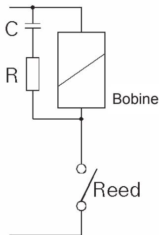
Alimentation Courant Alternatif
