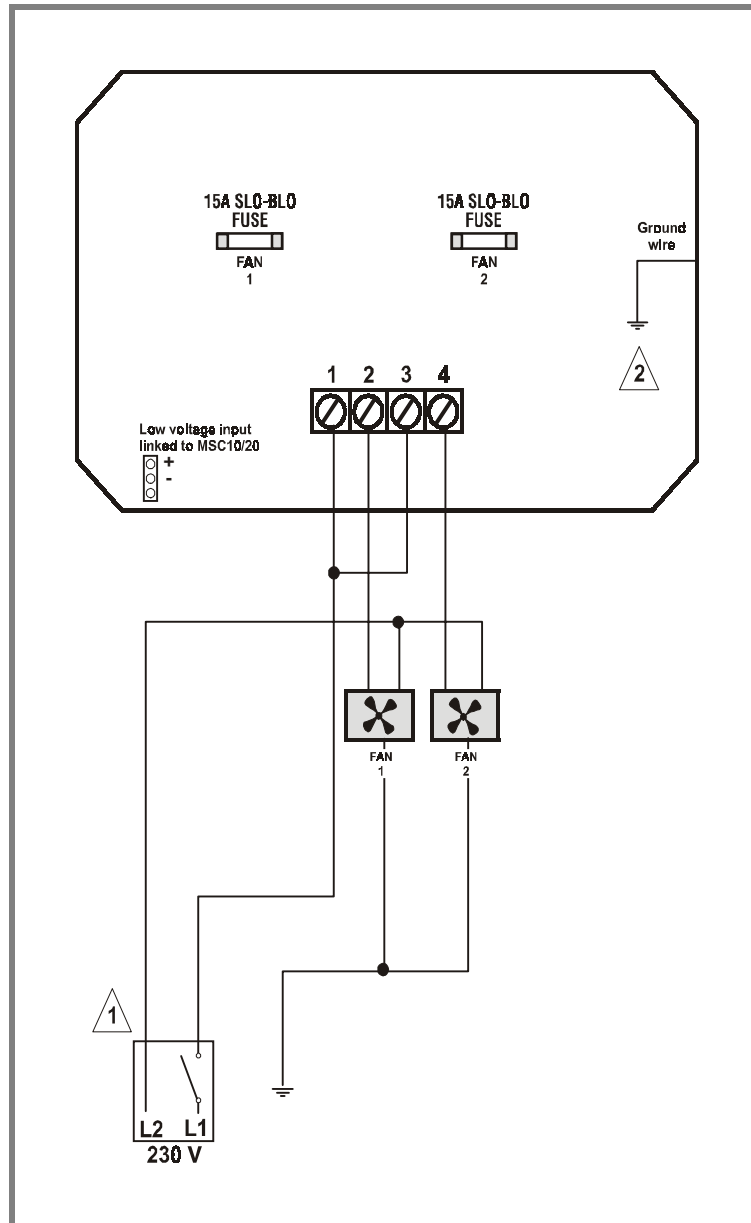
Fig. 2 Schéma de branchement des ventilateurs 230VAC.
