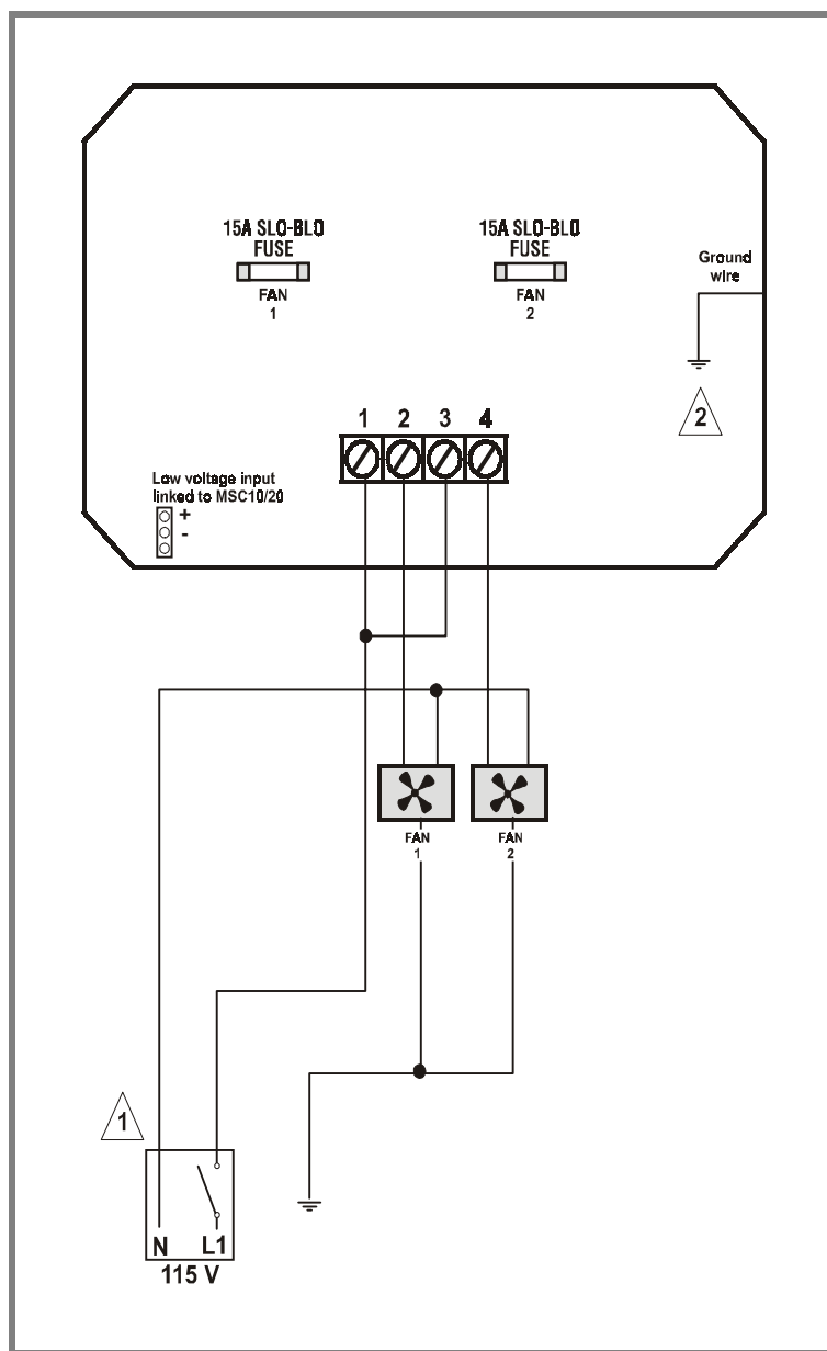
Fig. 1 Schéma de branchement des ventilateurs 115VAC.
