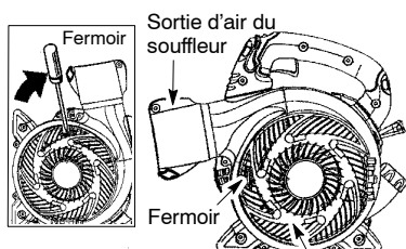
Couvercle d'arrivée d'air de l'aspirateur
