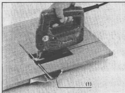
(1) Guide de gabarit
