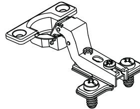
14H HINGE - 2
