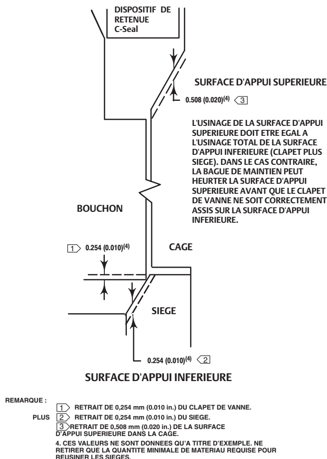
Figure 14. Exemple d'usinage de surfaces d'appui inférieures (clapet de vanne au siège) et supérieure (joint C-Seal à cage)
