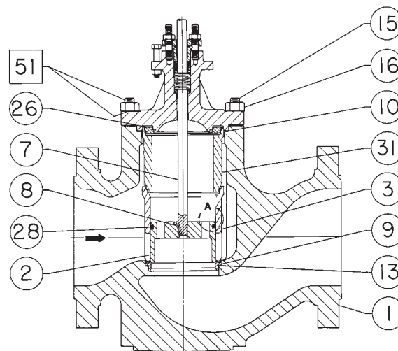
VANNE DE 12 X 8 NPS AVEC CAGE STANDARD
