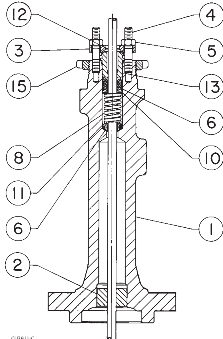
CHAPEAU A EXTENSION DE TYPE 1 OU 2
