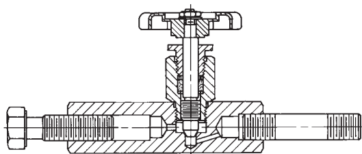
VANNE D'ISOLEMENT/DE LUBRIFICATION
