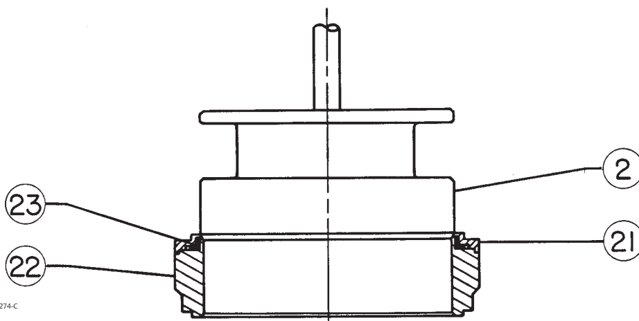
DETAIL DU SIEGE EN ELASTOMERE
