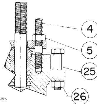
DETAIL DE LA VISSERIE DE L'ACTIONNEUR A BOSSAGE D'ARCADE DE 127 mm (5 in.)
