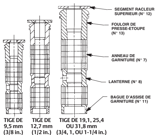
Figure 5. Détail des agencements de garniture en PTFE/composite
