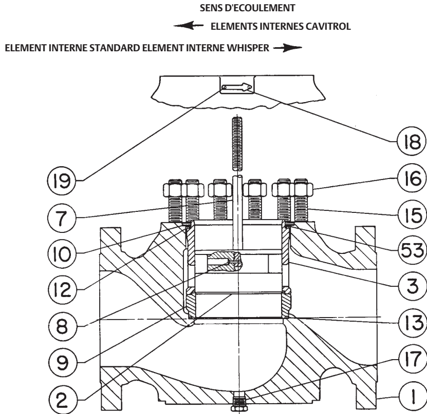
VANNE COMPLETE AVEC SIEGE EN METAL ET BOUCHON DE PURGE EN OPTION
