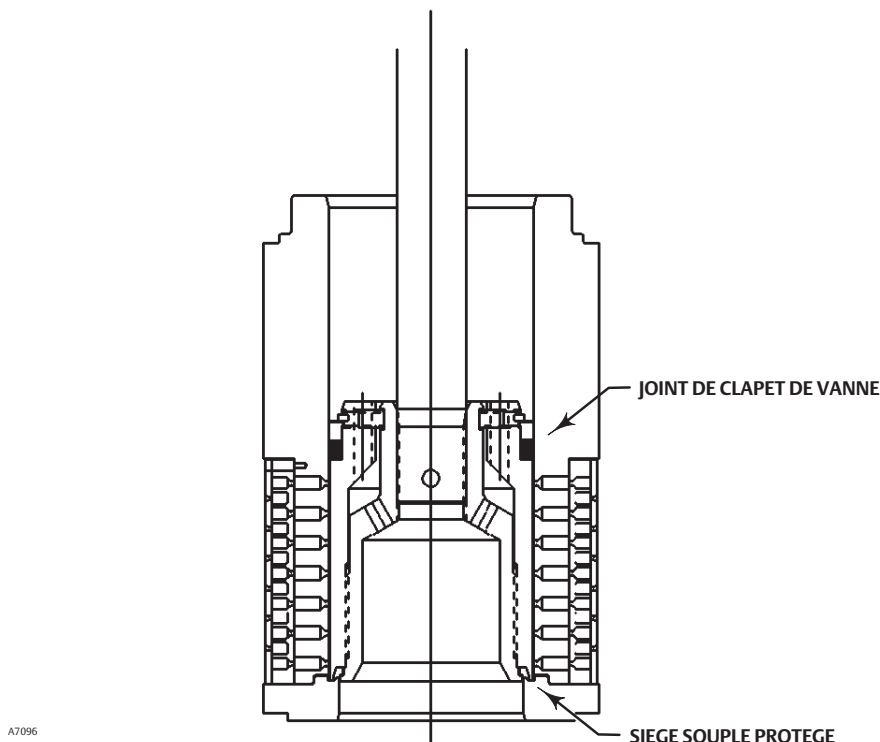
Figure 8. Eléments internes à fermeture étanche (TSO) équilibrés types
