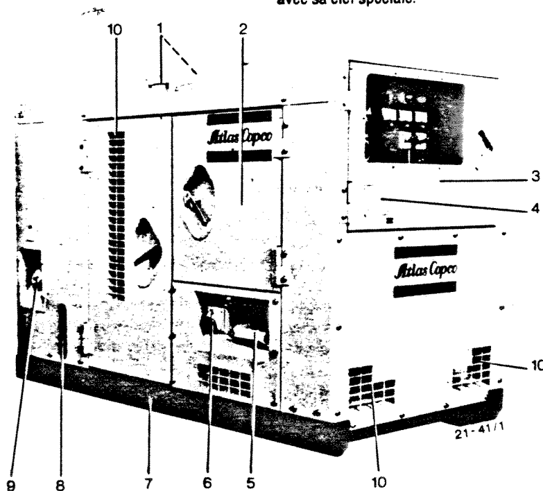
Fig. 2. QAS40
