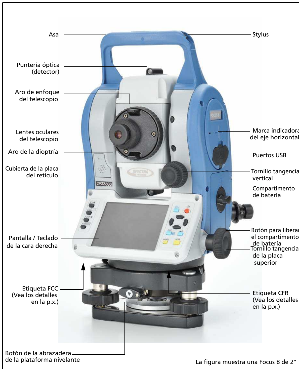
Figura 1.1 Estación total de la serie Focus 8 – Cara derecha
