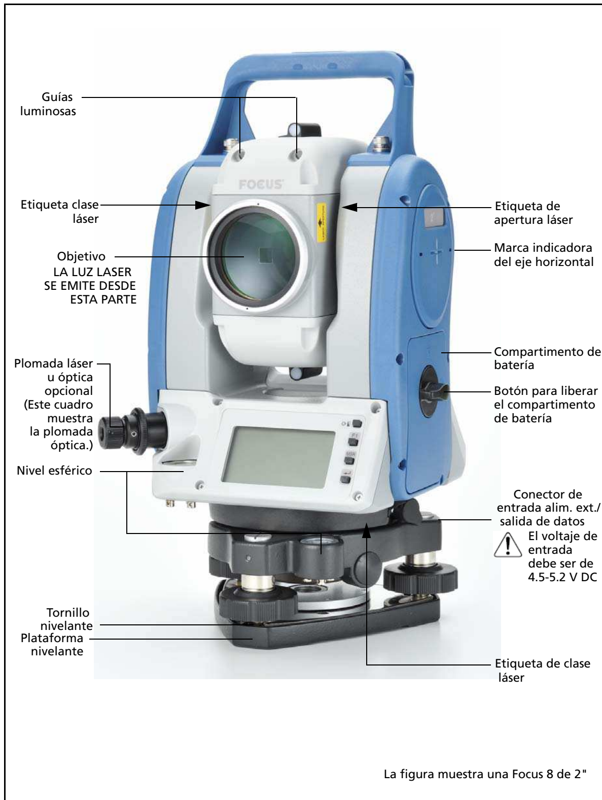
Figura 1.2 Estación total de la serie Focus 8 – Cara izquierda
