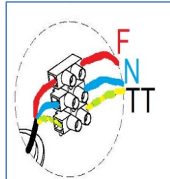
Figura 3 (Conexión eléctrica)
