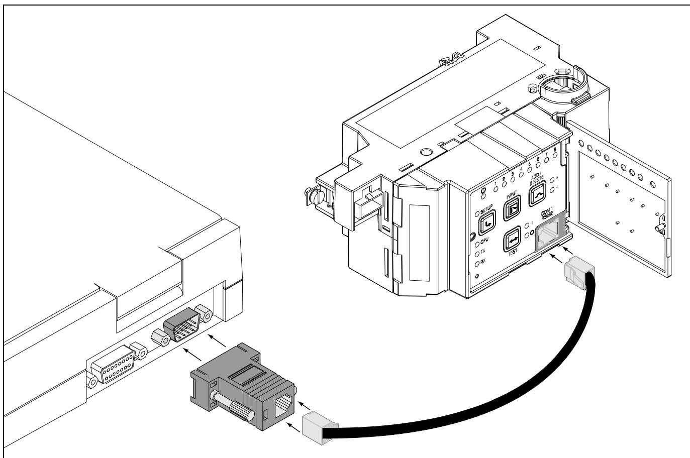
Figura 1: Conexión del cable en serie del panel frontal del controlador
